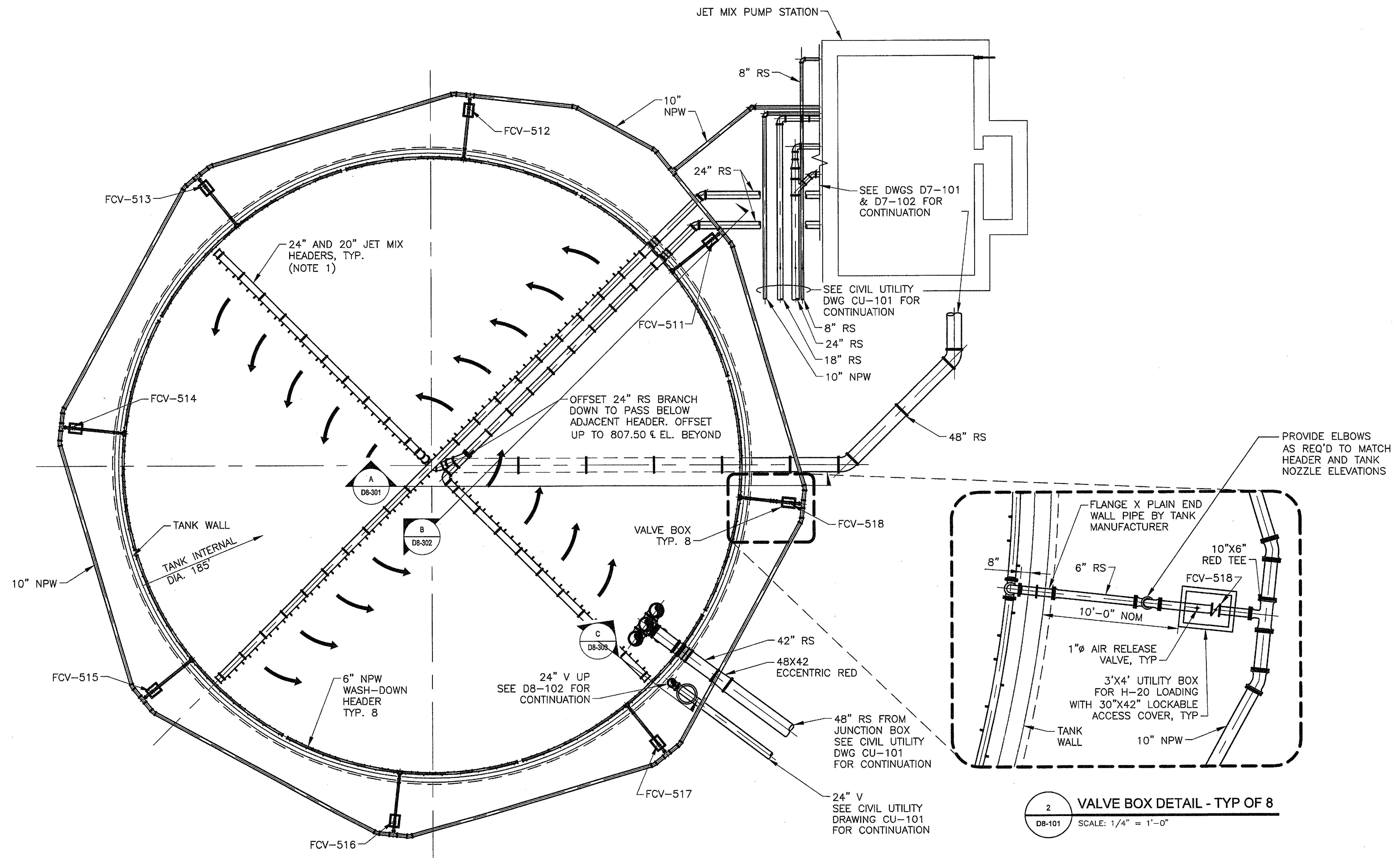
1 BASE PLAN D8-101 SCALE: 1/16" = 1'-0"
