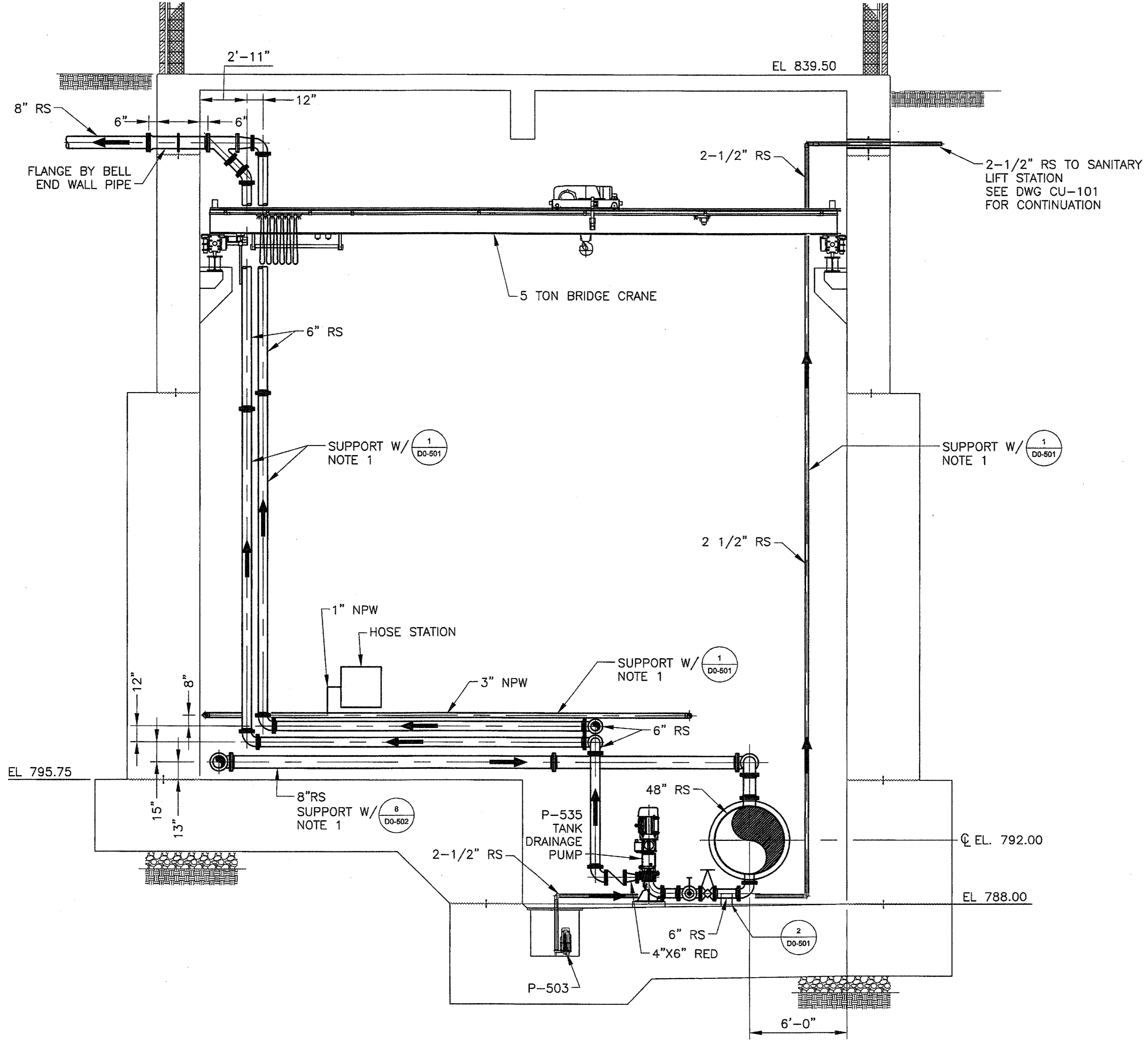
E SECTION E D7-305 SCALE: 1/4" = 1'-0"
