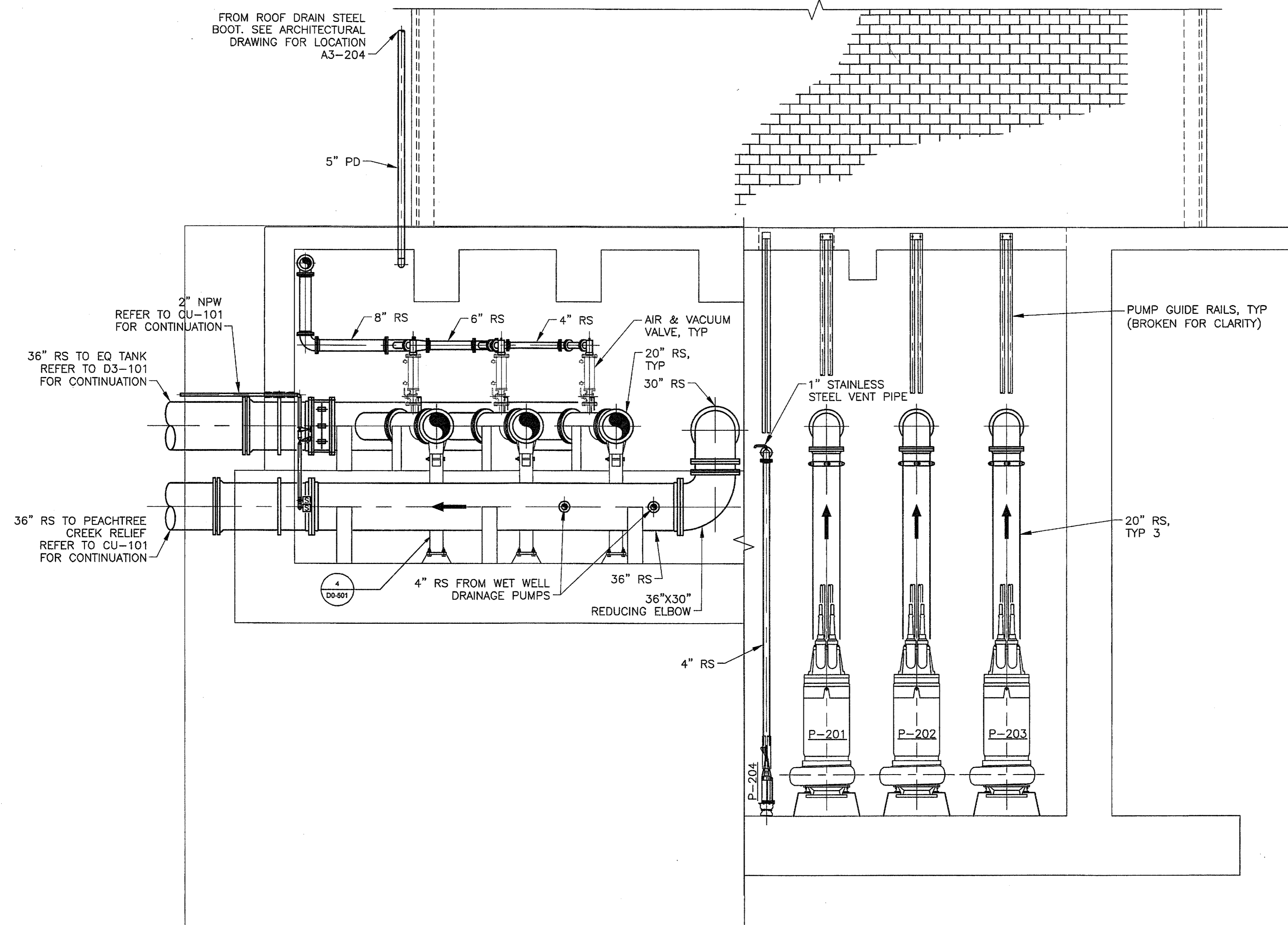
D SECTION D D3-304 SCALE: 1/4" = 1'-0"
