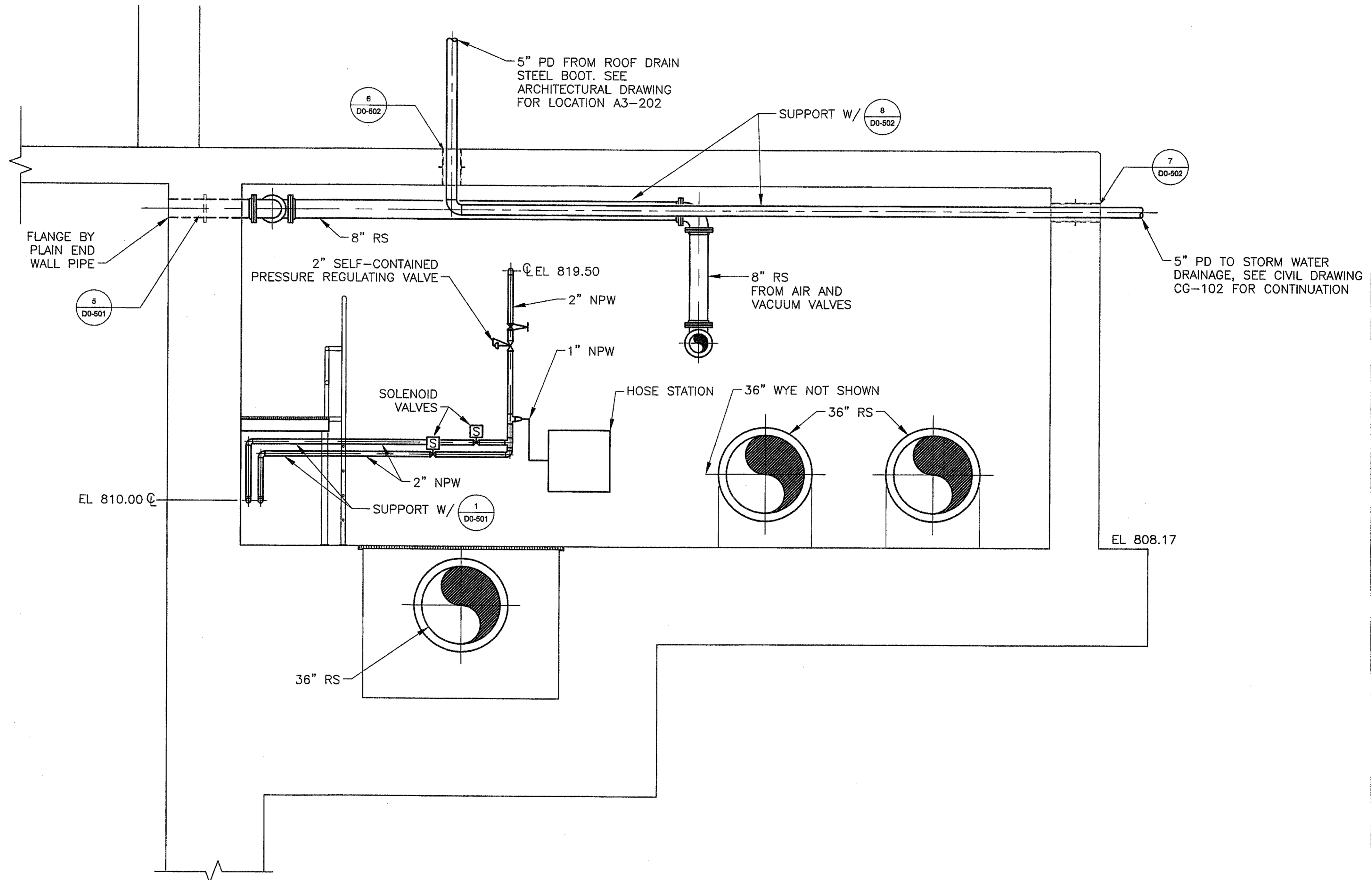
SECTION C D3-303 SCALE: 3/8" = 1'-0"
