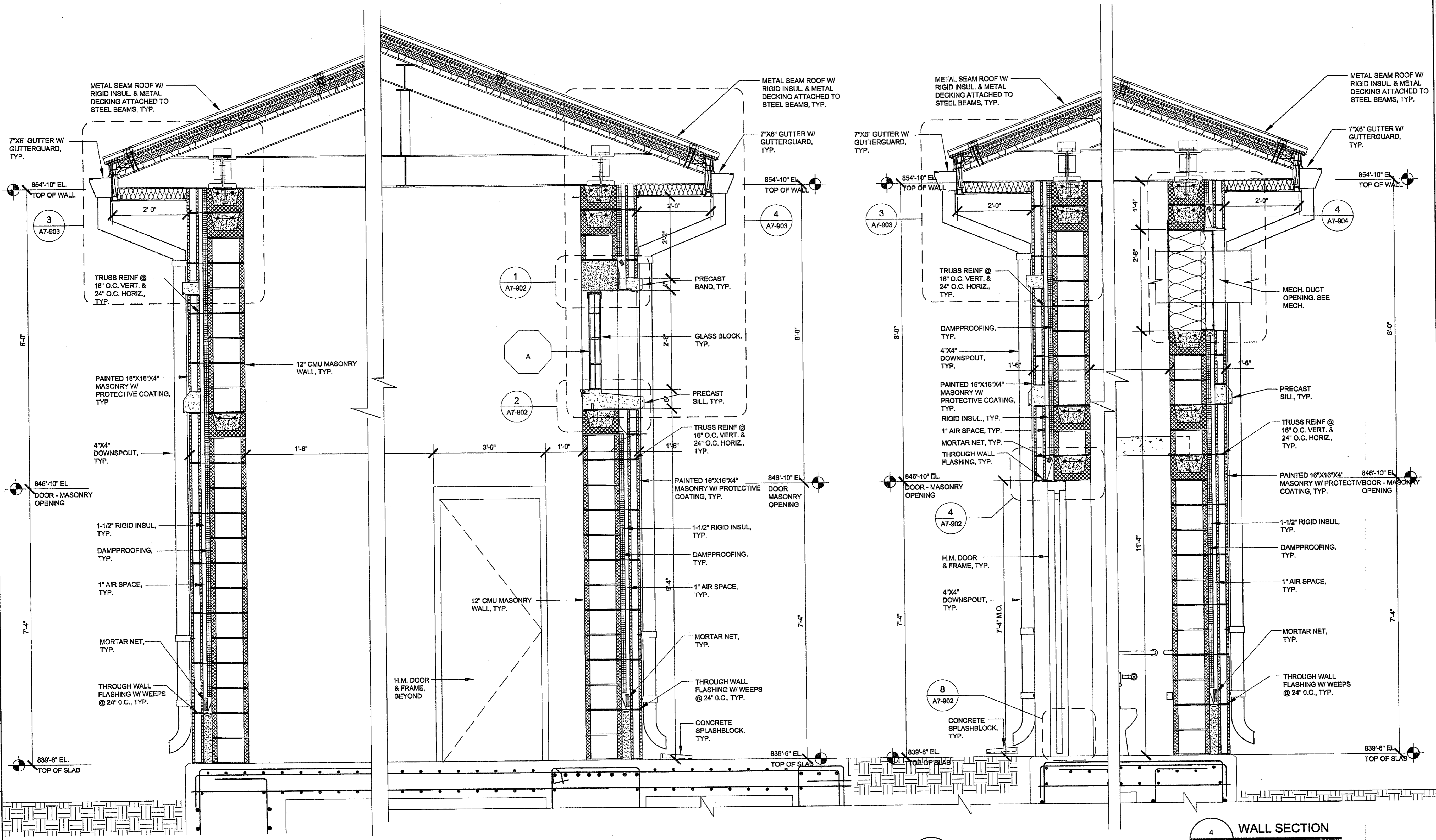
1 WALL SECTION A7-701 SCALE: 3/4"=1'-0"
