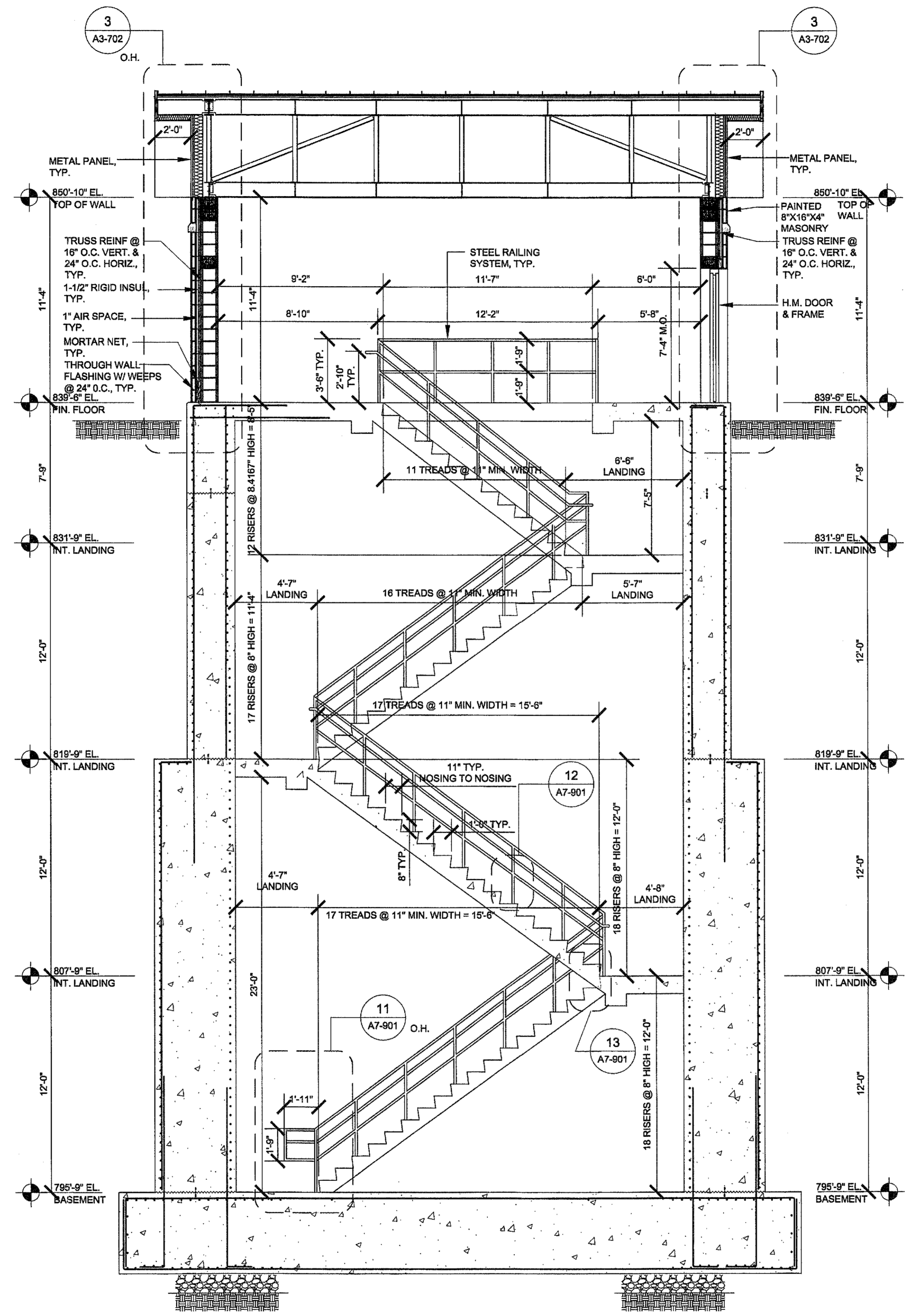
1 STAIR SECTION A7-304 SCALE: 1/4" = 1'-0"
