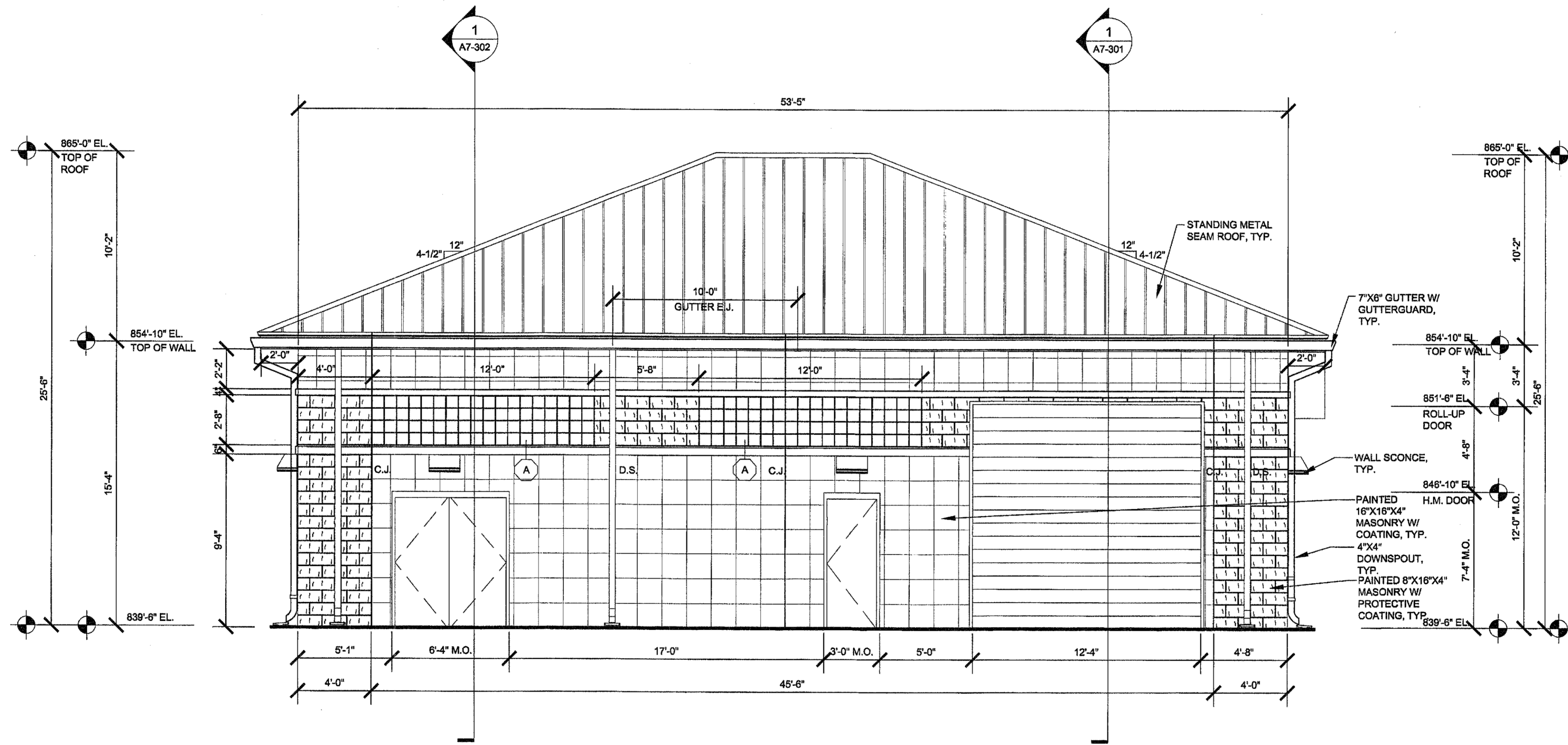
1 ELEVATION A7-204 SCALE: 1/4" = 1'-0"
