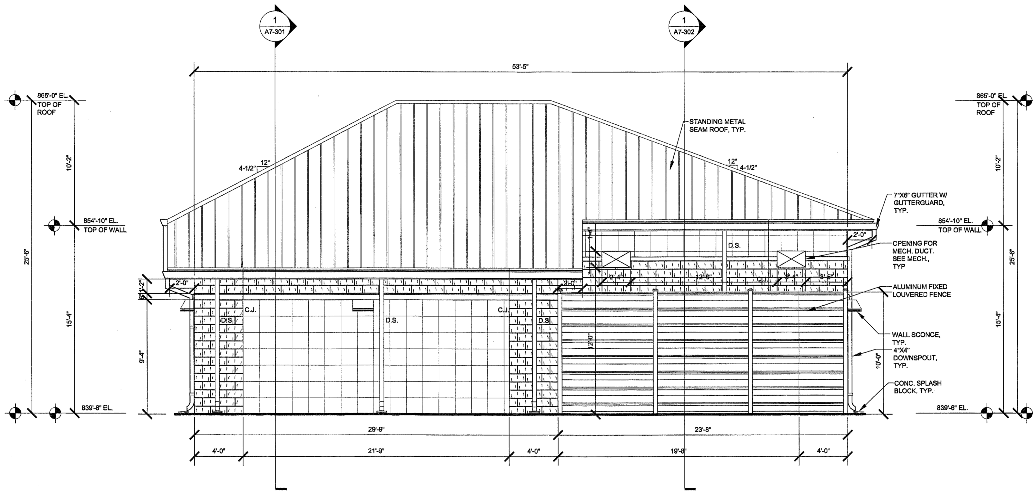
1 ELEVATION A7-203 SCALE: 1/4" = 1'-0"
