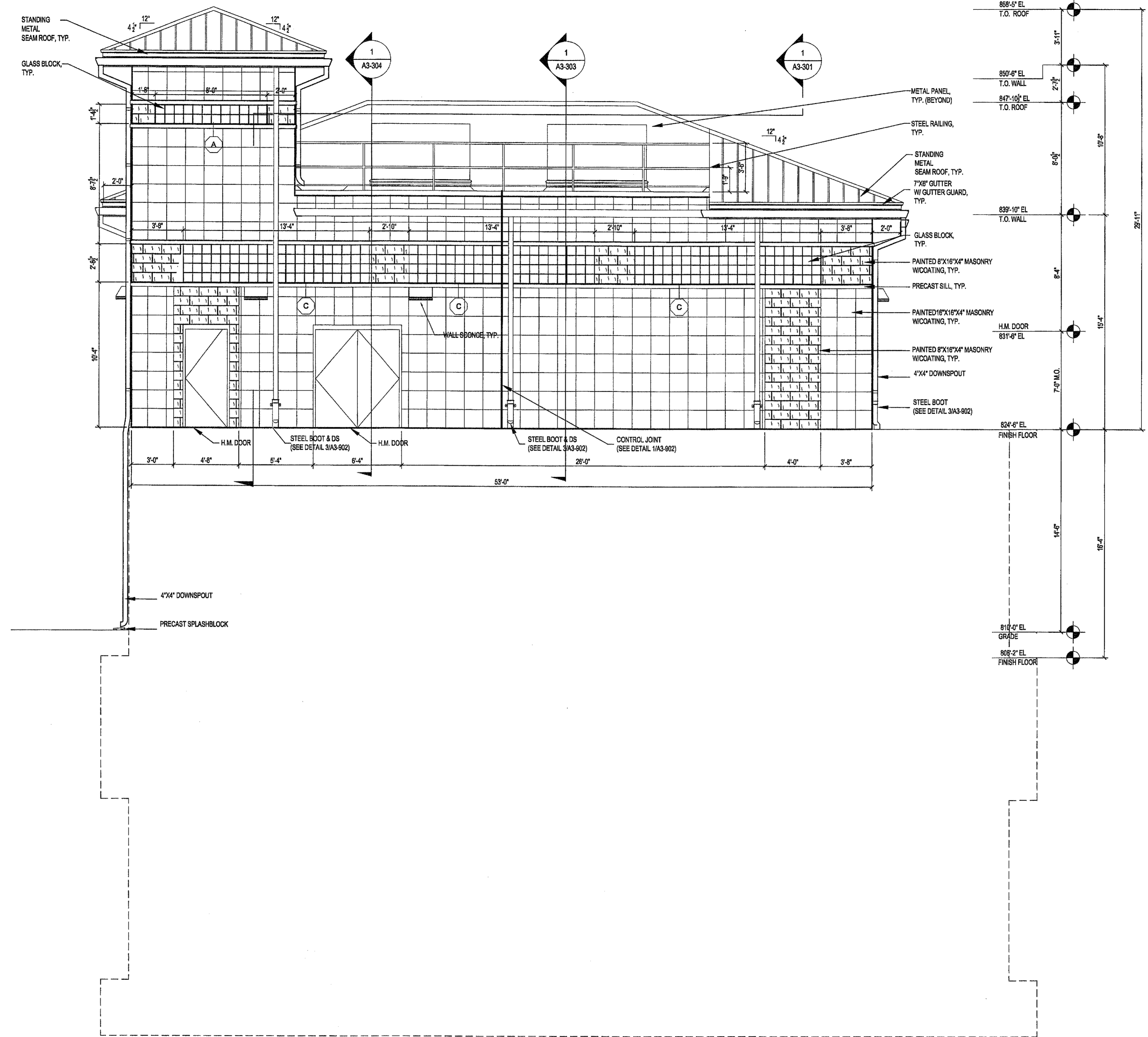
1 NORTH ELEVATION A3-201 SCALE: 1/4" = 1'-0"
