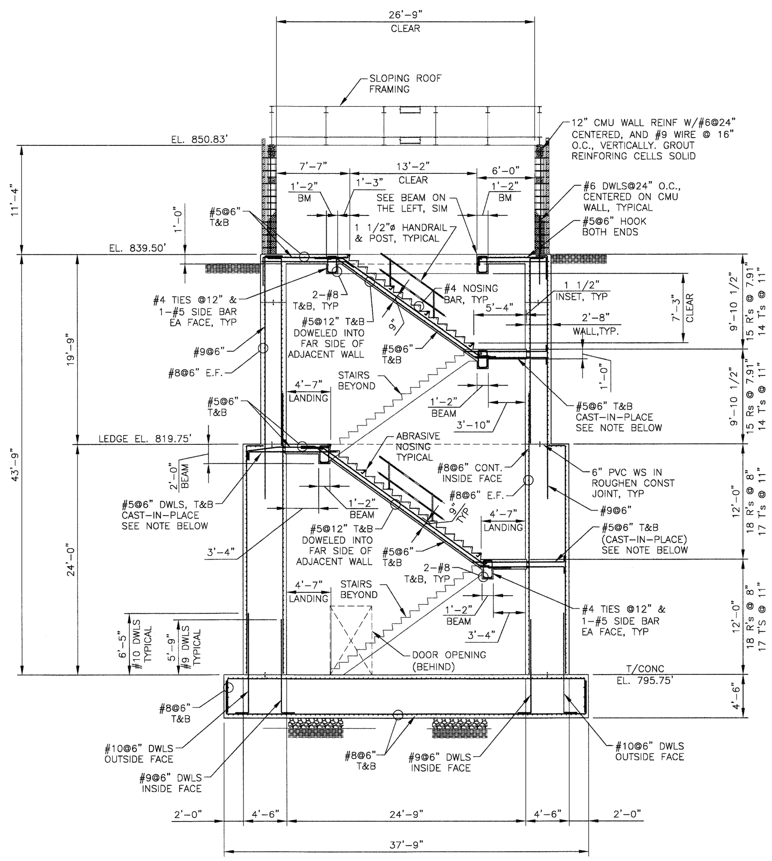
E SECTION 97-305 SCALE: 3/16" = 1'-0"
