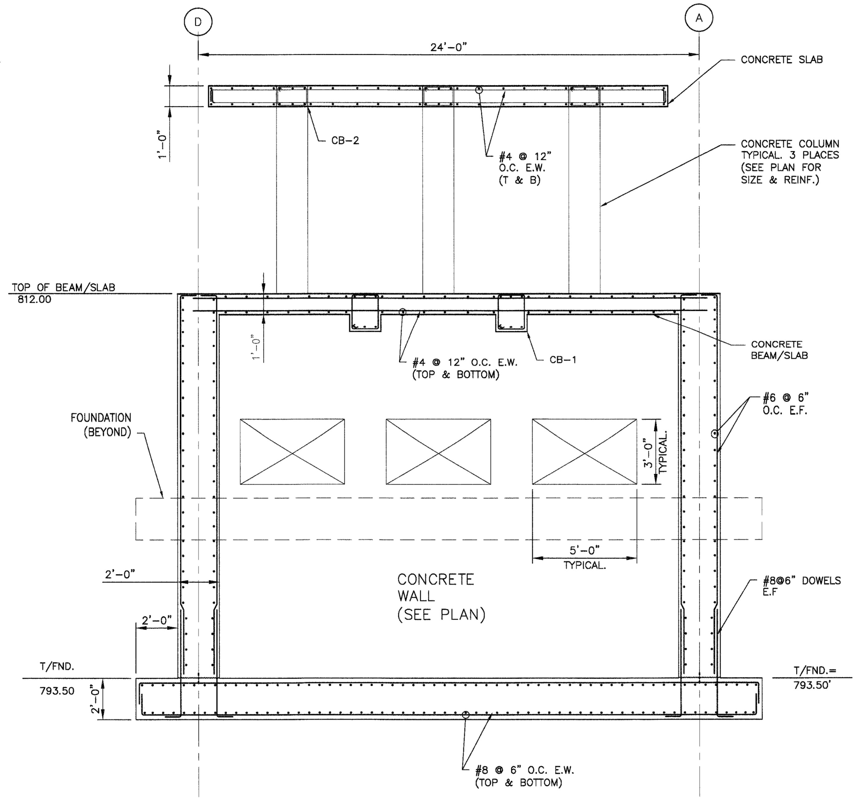
A SECTION S2-303 SCALE: 3/8" = 1'-0"
