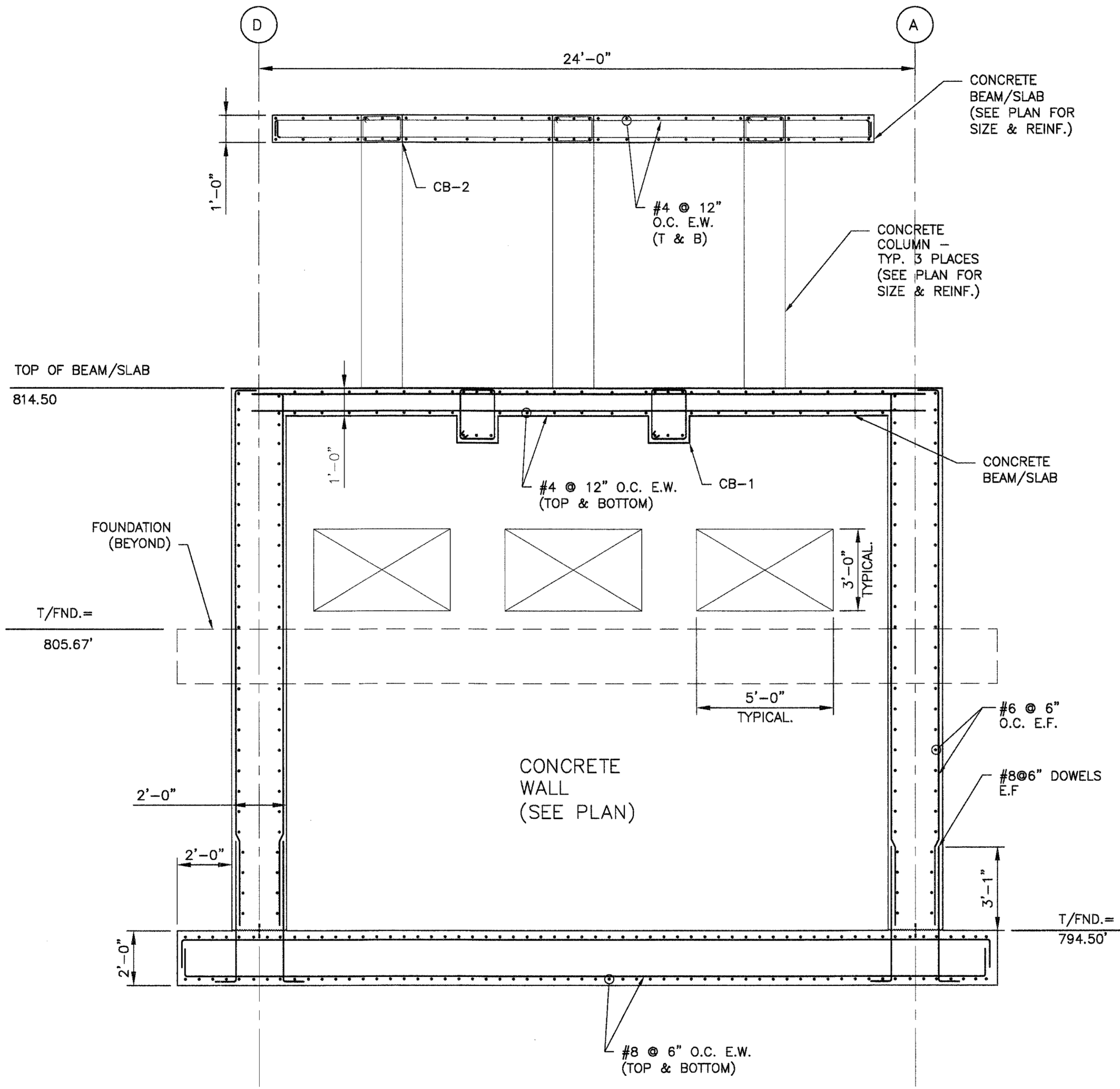
A SECTION S1-303 SCALE: 3/8" = 1'-0"
