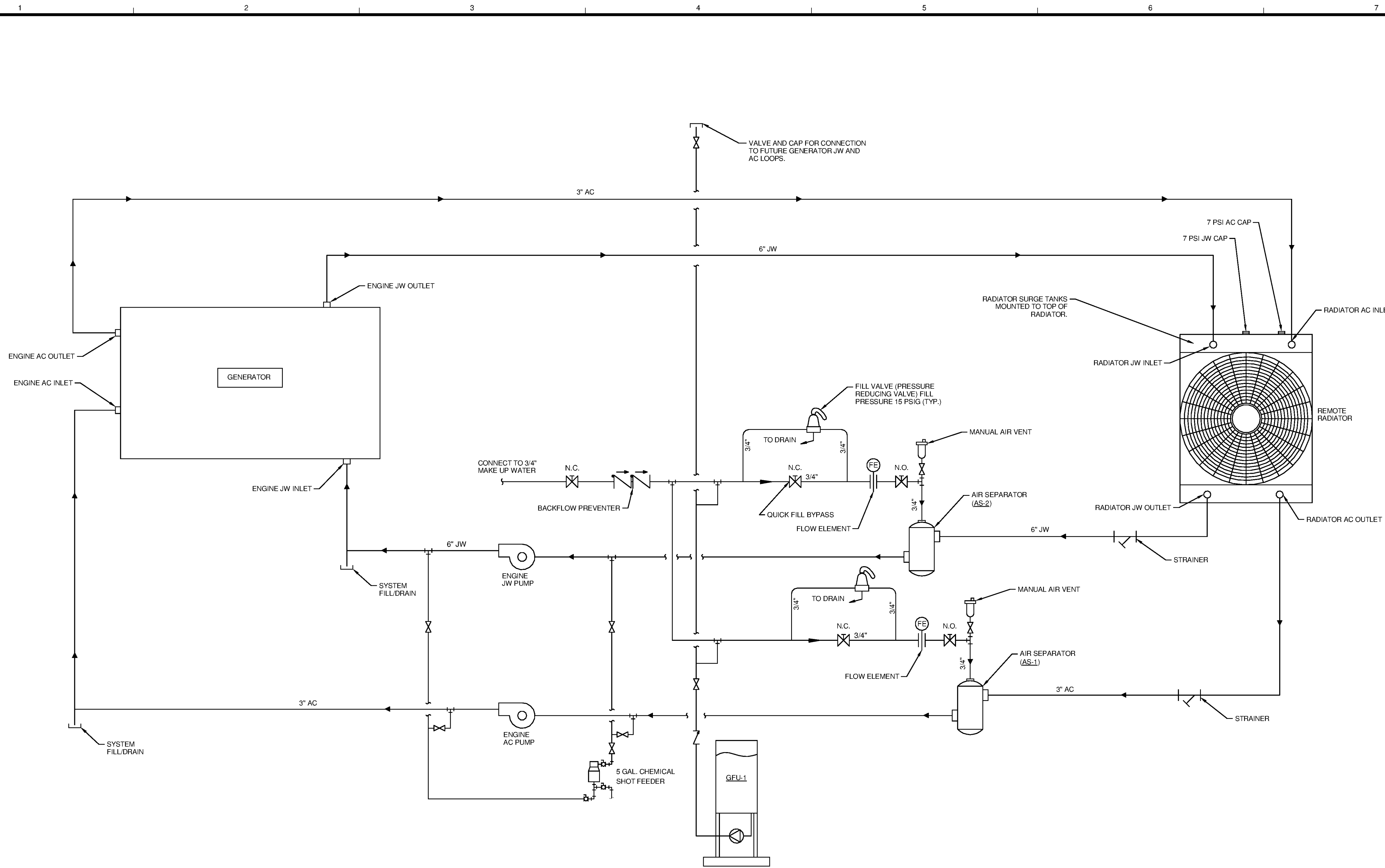
1 GENERATOR COOLING SCHEMATIC SCALE: N.T.S.
