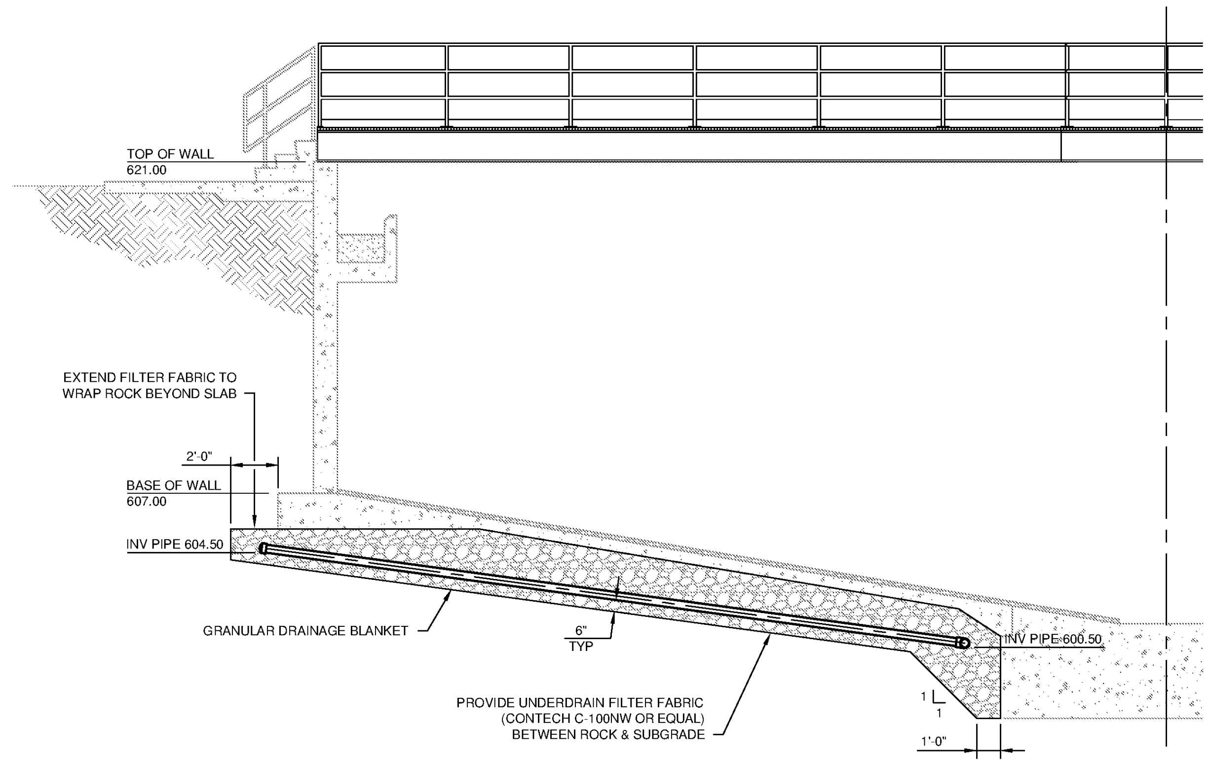
SECTION A D-5101 SCALE: 1/4"=1'-0"
