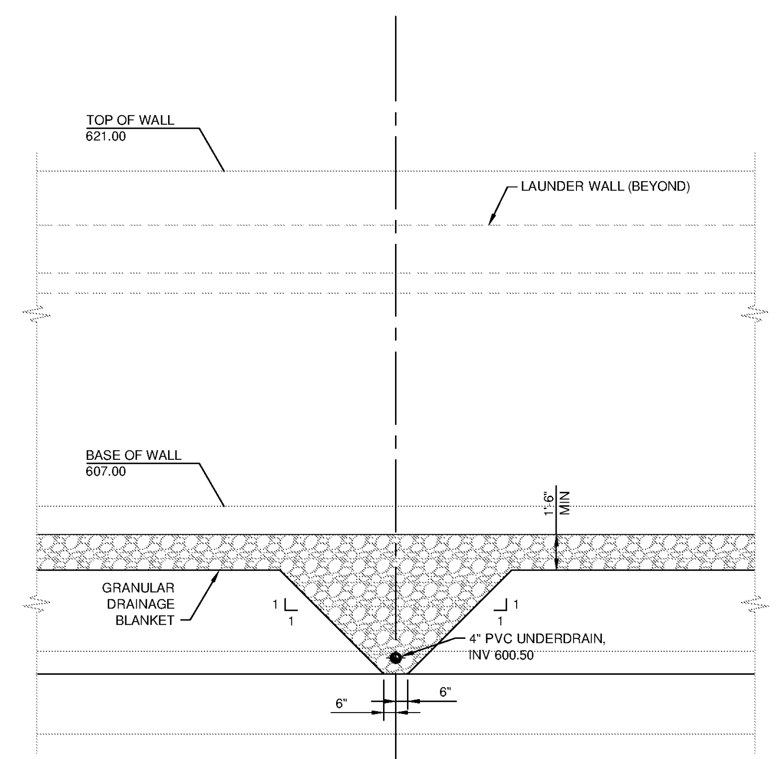
SECTION A D-5101 SCALE: 1/4"=1'-0"
