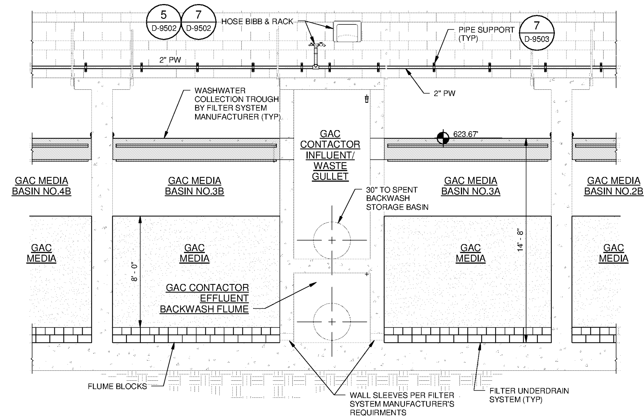
H SECTION D-3101 SCALE: 1/4" = 1'-0"
