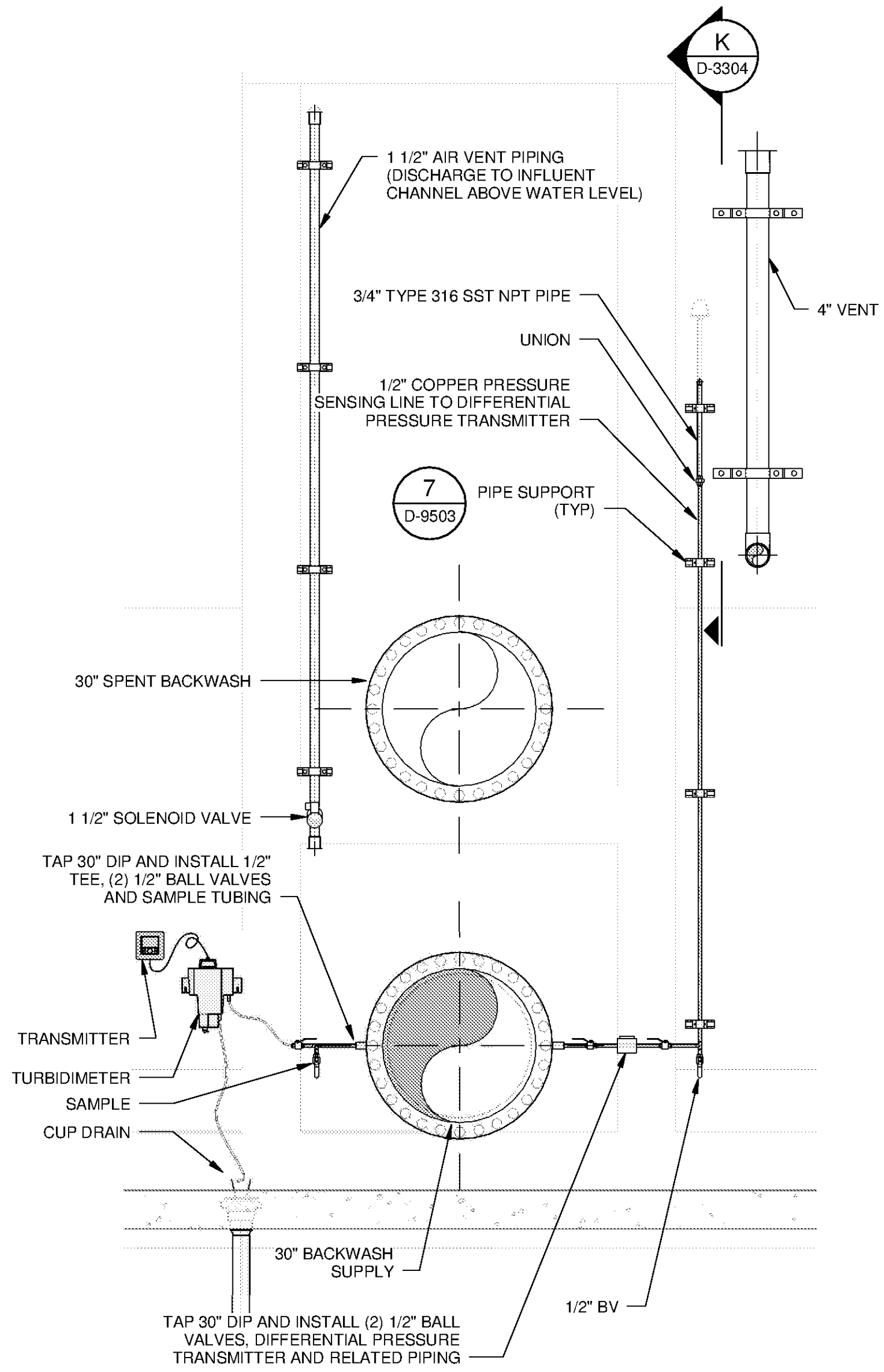
J SECTION D-3302 SCALE: 1/2" = 1'-0"
