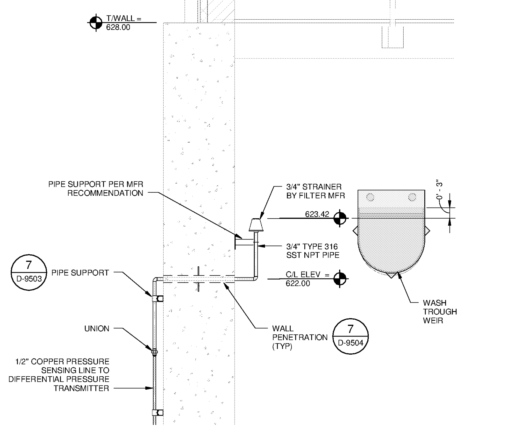
K SECTION D-3304 SCALE: 3/4" = 1'-0"
