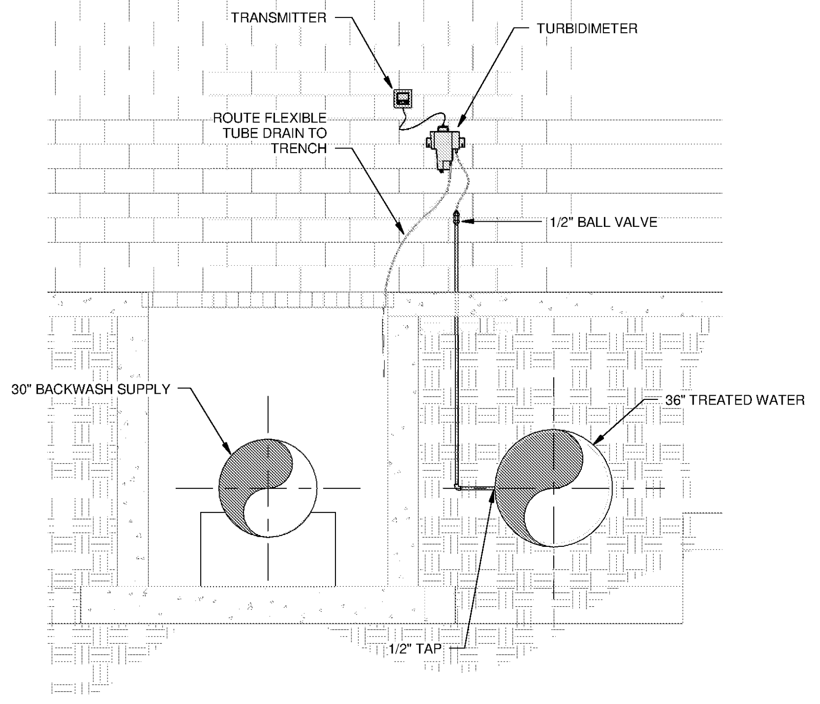
L SECTION D-3101 SCALE: 3/8" = 1'-0"
