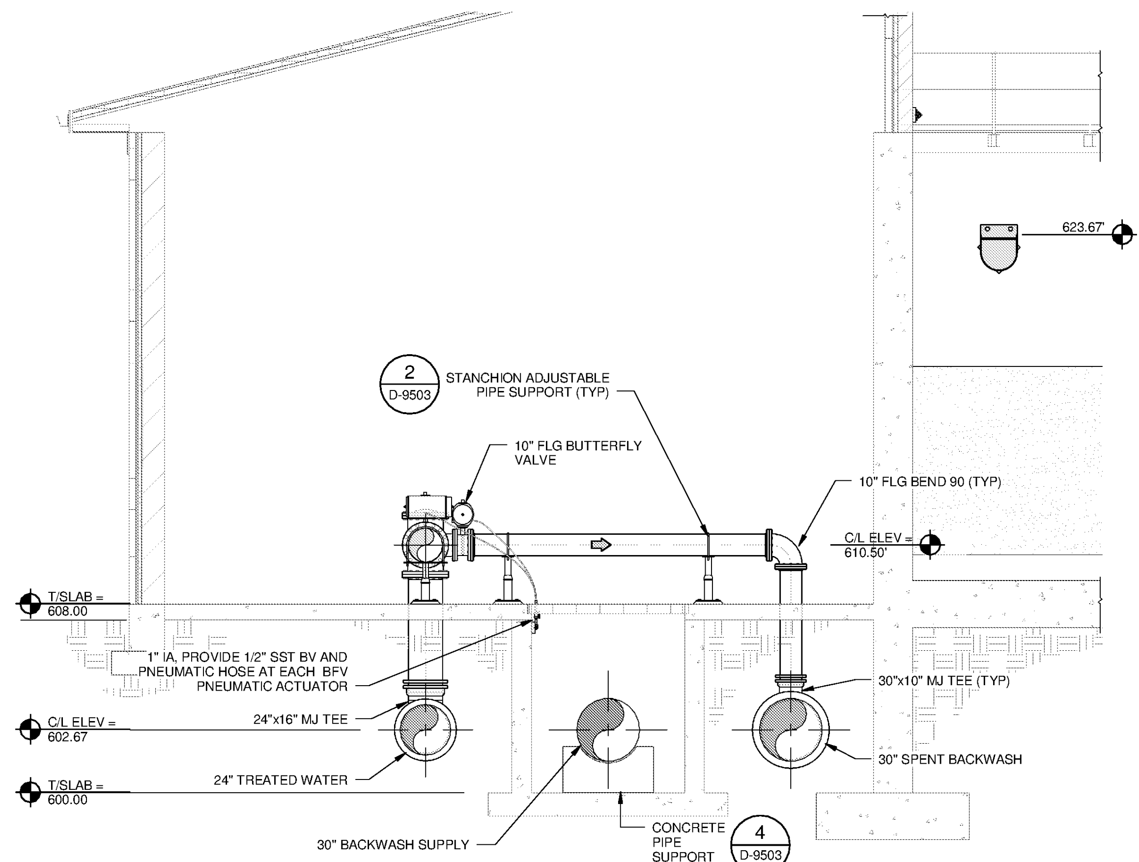
G SECTION D-3101 SCALE: 1/4" = 1'-0"
