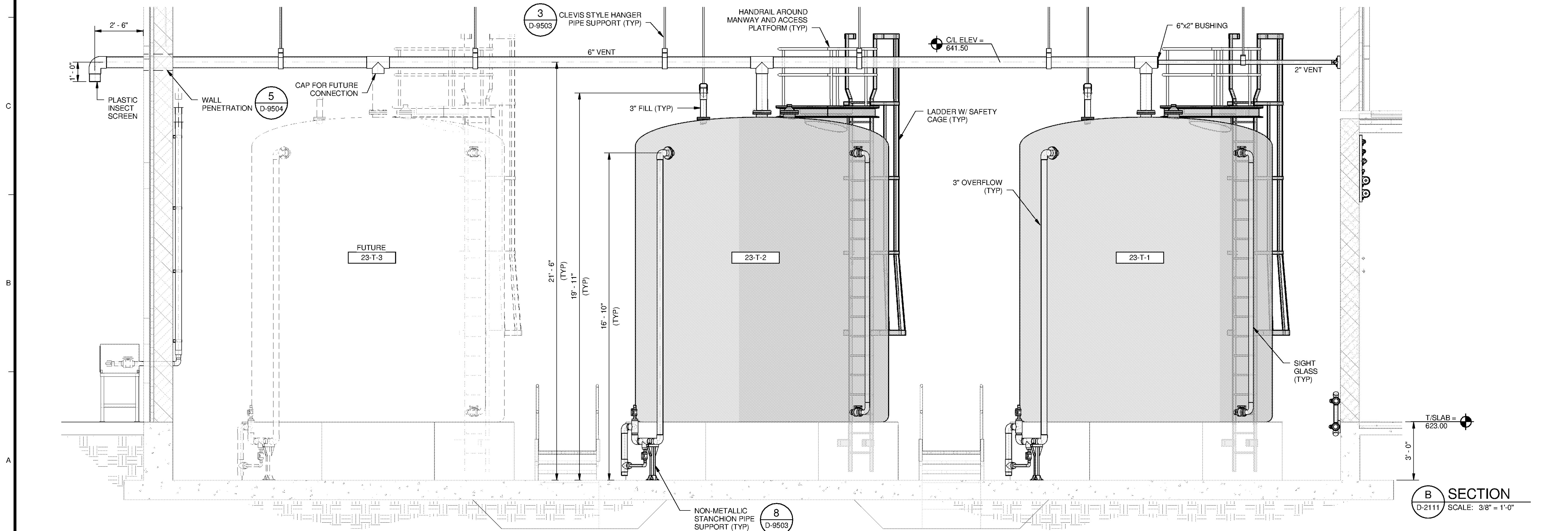
A SECTION D-2111 SCALE: 3/8" = 1'-0"
