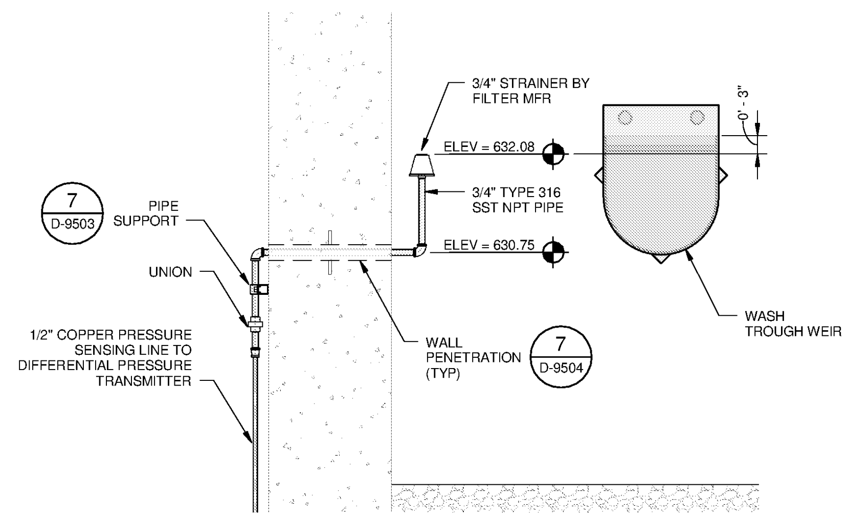
K SECTION D-2306 SCALE: 3/4" = 1'-0"
