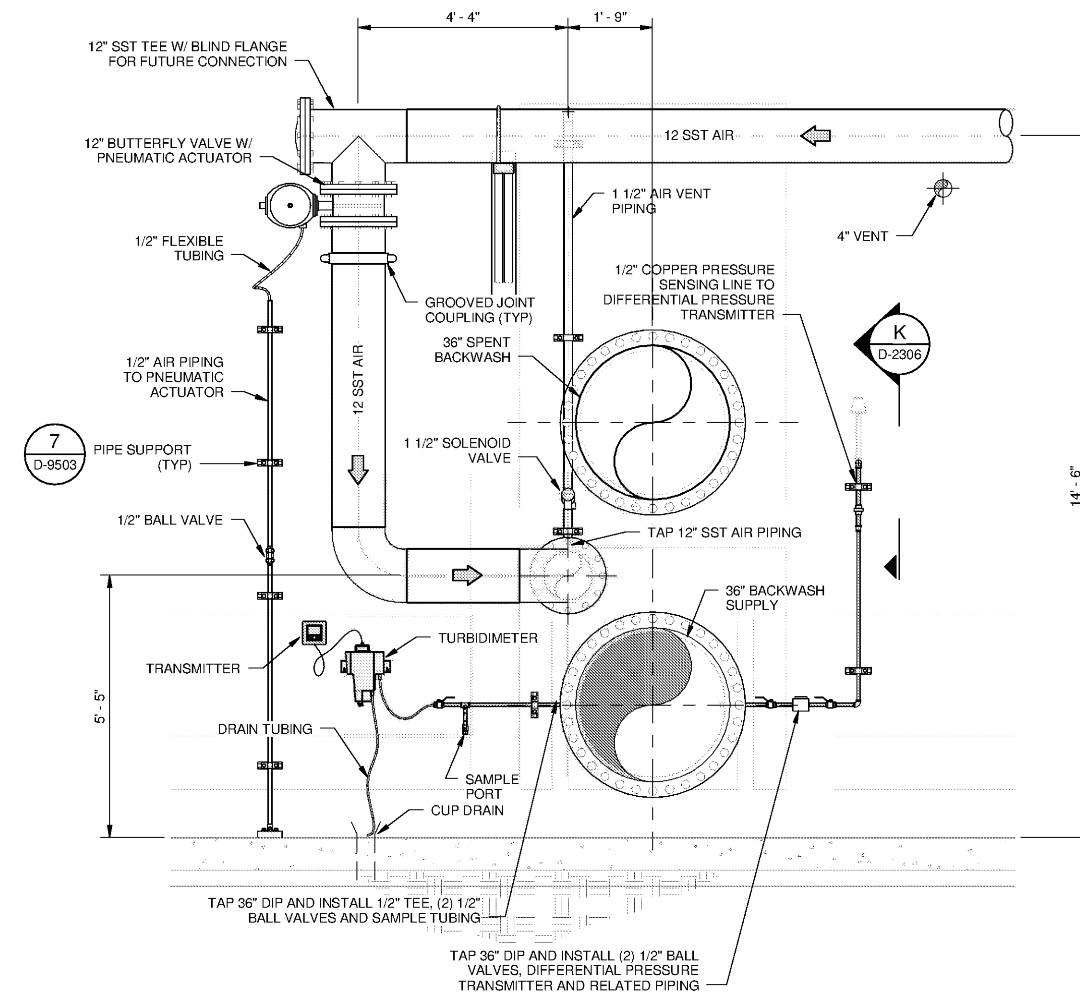
J SECTION D-2304 SCALE: 1/2" = 1'-0"
