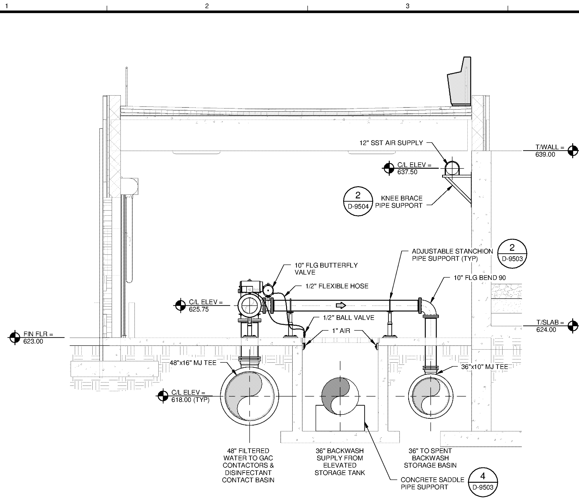
G SECTION D-2106 SCALE: 1/4" = 1'-0"
