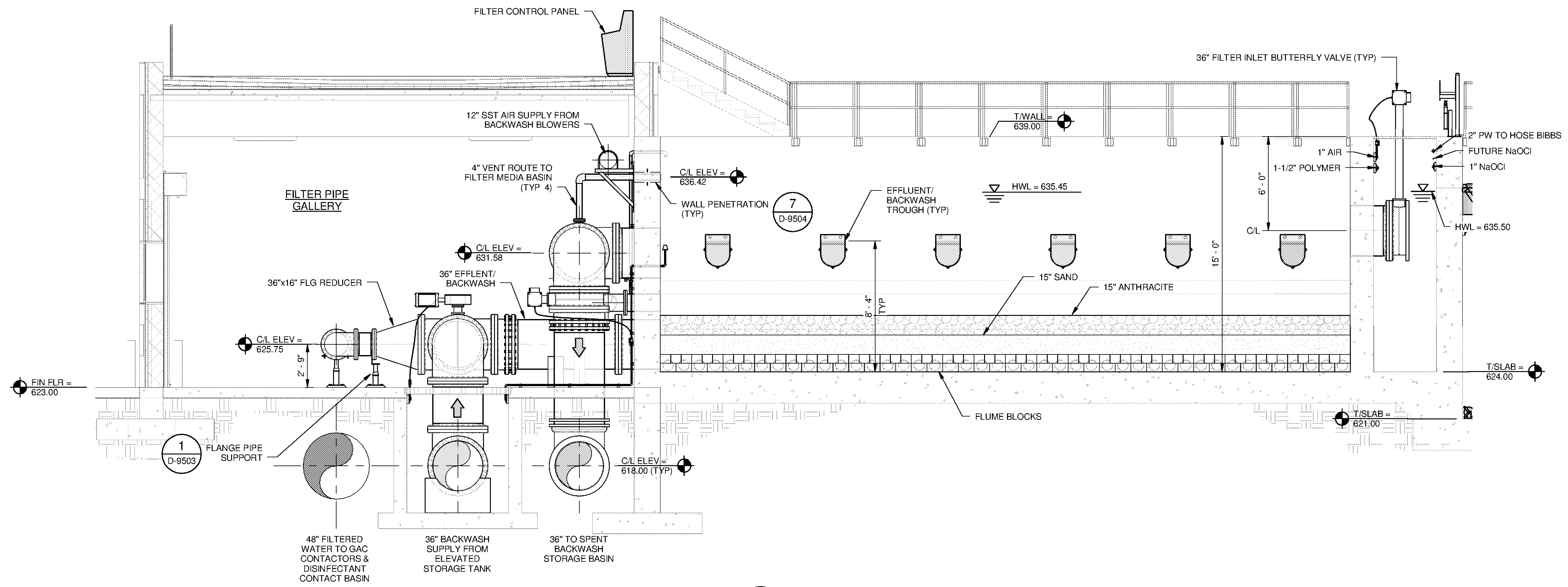
E SECTION D-2106 SCALE: 1/4" = 1'-0"
