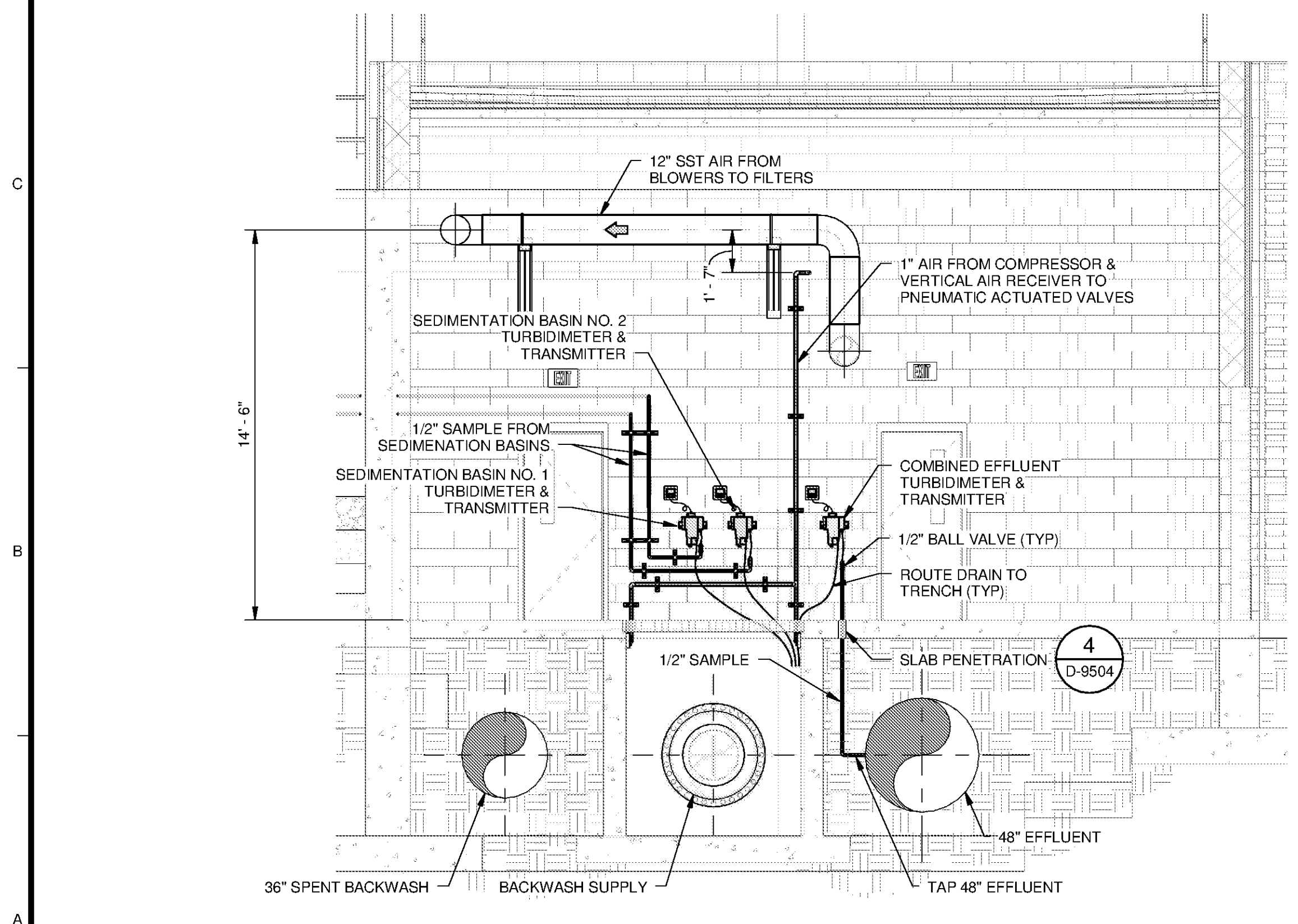
D SECTION D-2106 SCALE: 1/4" = 1'-0"
