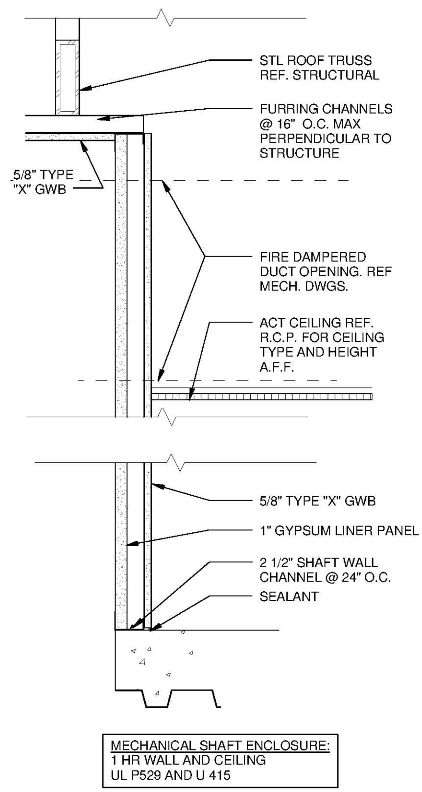
12 WALL TYPE 12 SCALE: 1 1/2" = 1'-0"
