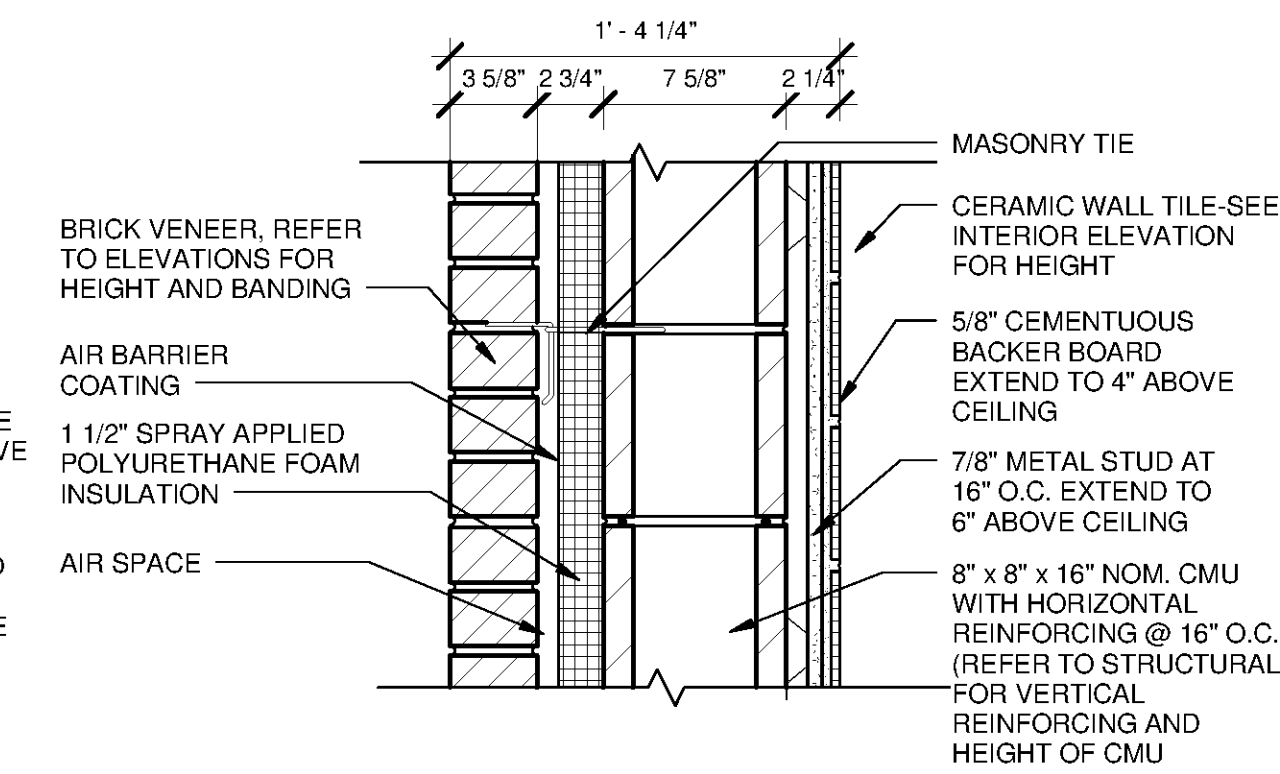
5 WALL TYPE 5 SCALE: 1 1/2" = 1'-0"
