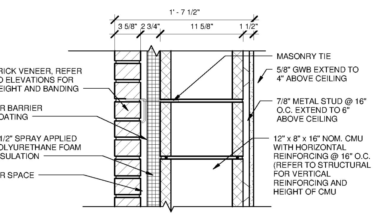
4 WALL TYPE 4 SCALE: 1 1/2" = 1'-0"
