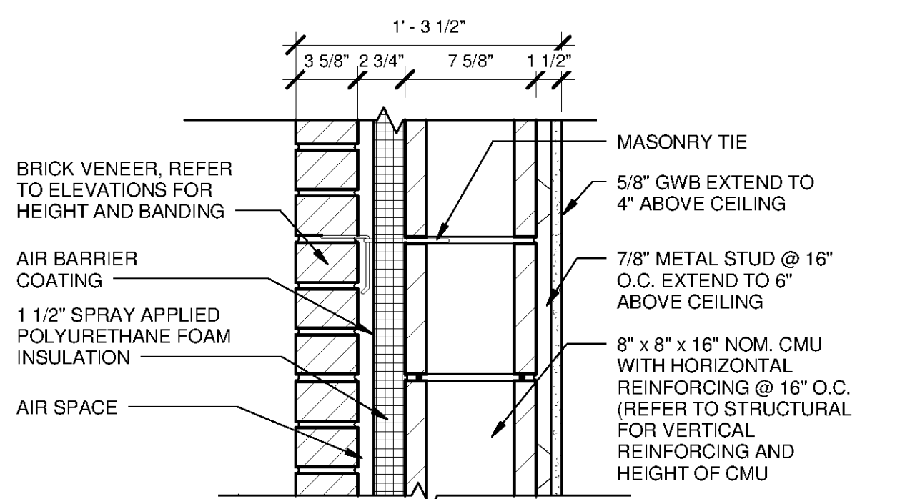
3 WALL TYPE 3 SCALE: 1 1/2" = 1'-0"
