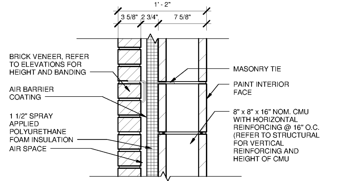
1 WALL TYPE 1 SCALE: 1 1/2" = 1'-0"
