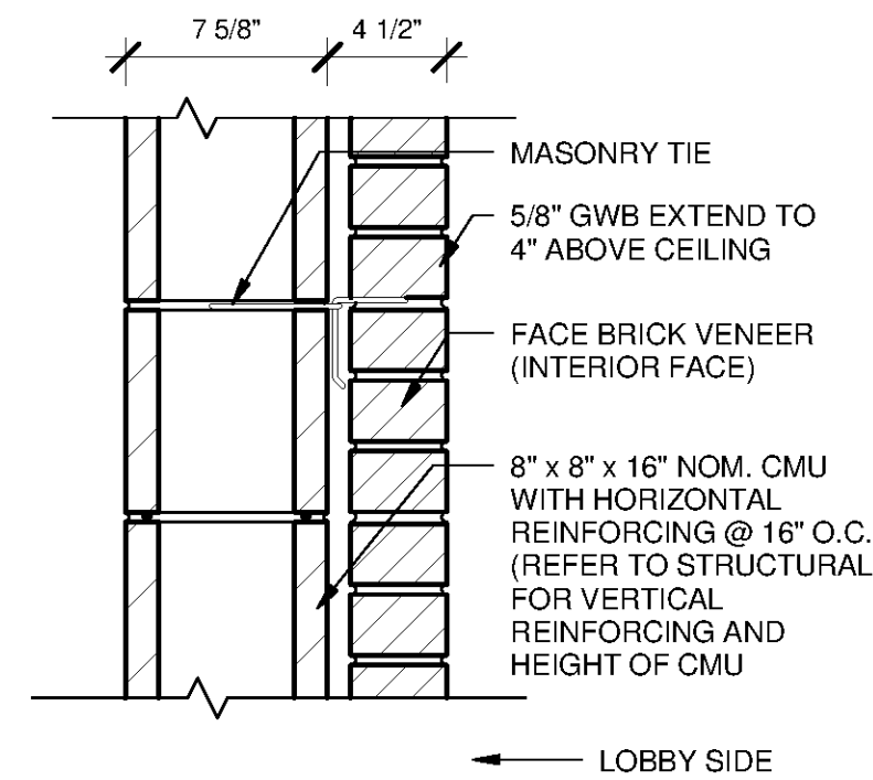
6 WALL TYPE 6 SCALE: 1 1/2" = 1'-0"
