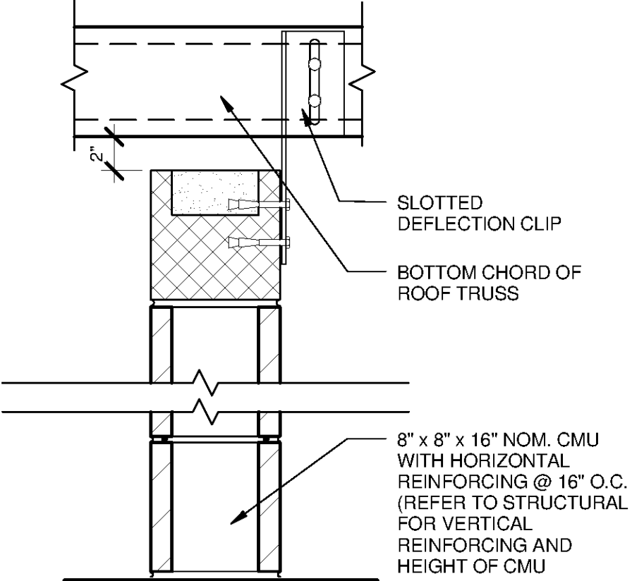
8 WALL TYPE 8 SCALE: 1 1/2" = 1'-0"
