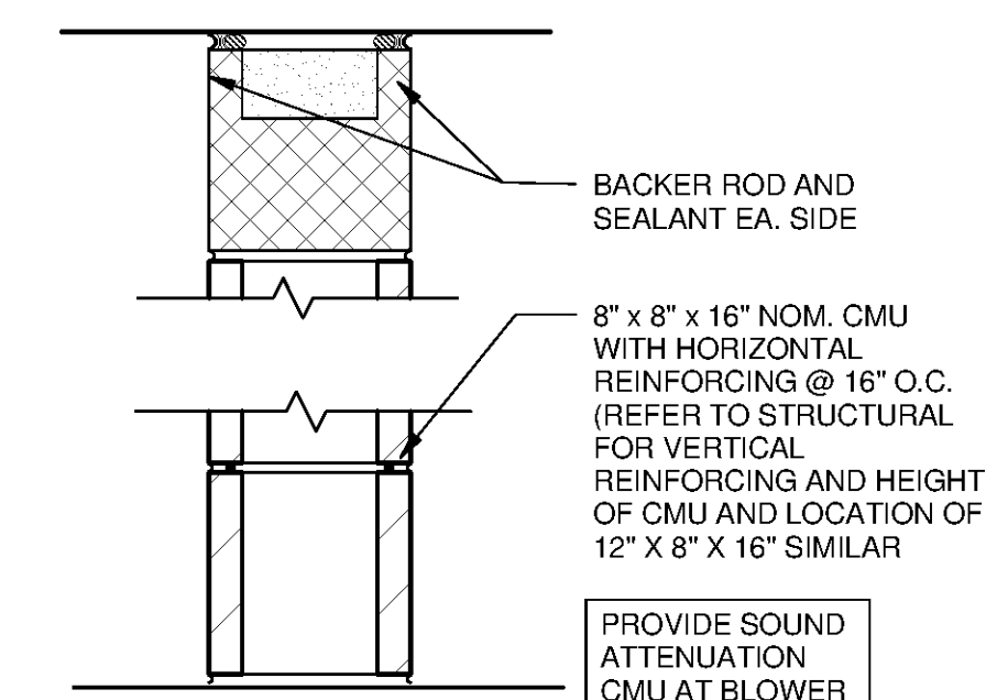
7 WALL TYPE 7 SCALE: 1 1/2" = 1'-0"
