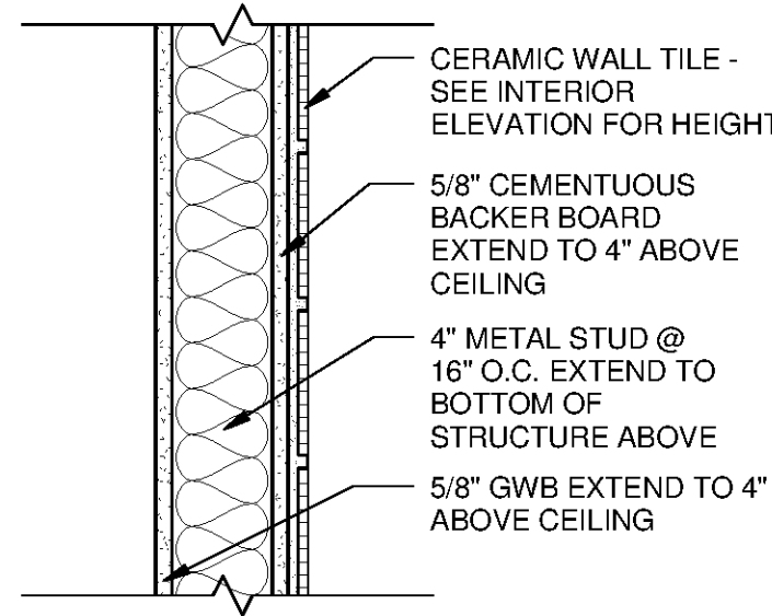
10 WALL TYPE 10 SCALE: 1 1/2" = 1'-0"
