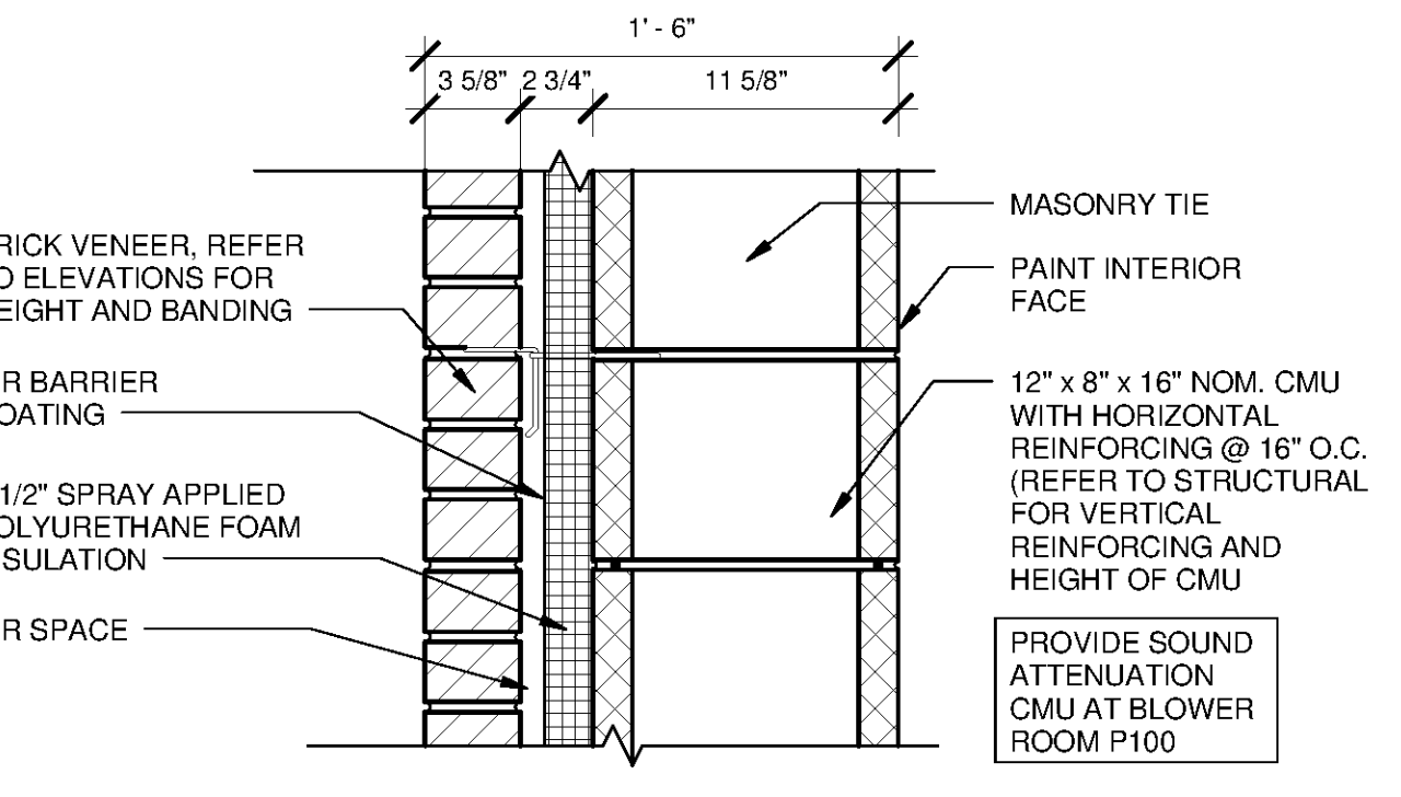
2 WALL TYPE 2 SCALE: 1 1/2" = 1'-0"
