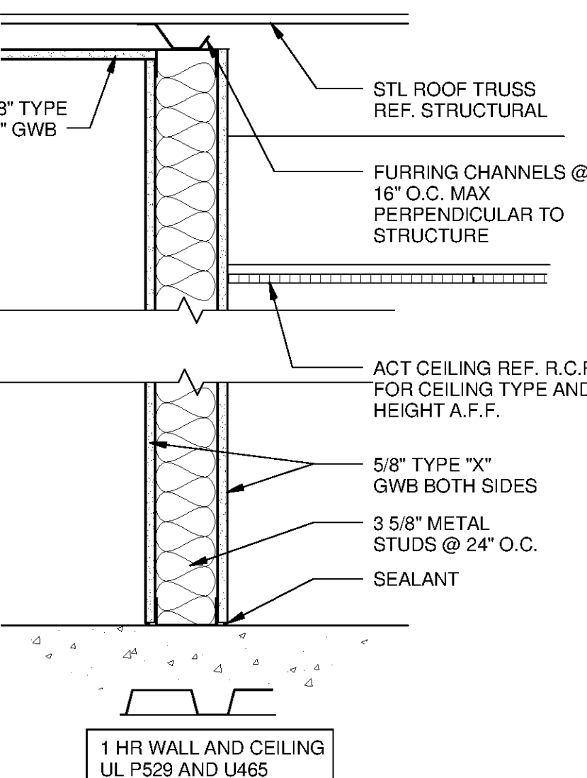
11 WALL TYPE 11 SCALE: 1 1/2" = 1'-0"
