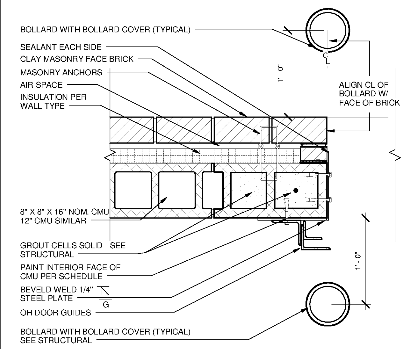
12 DOOR HEAD TYPE OH.1 A-3302 SCALE: 1 1/2" = 1'-0"
