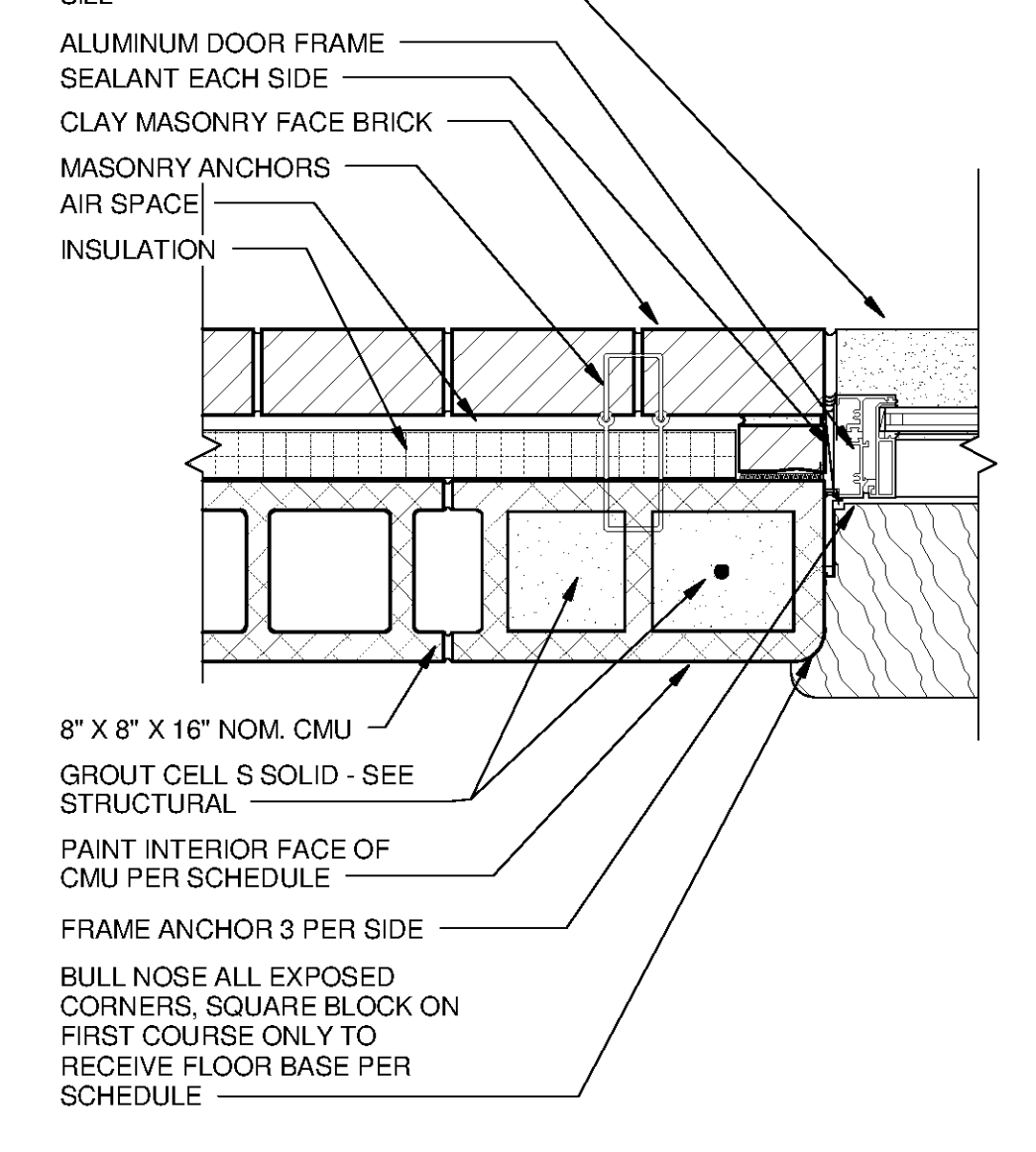
10 WINDOW JAMB TYPE WJ-A A-3102 SCALE: 1 1/2" = 1'-0"
