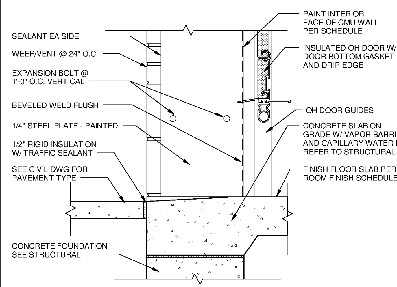
14 DOOR SILL TYPE OH.1 SCALE: 1 1/2" = 1'-0"
