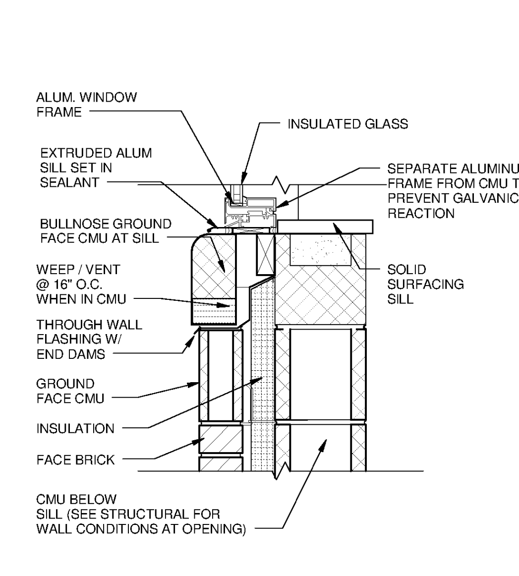
8 WINDOW SILL TYPE WS-A SCALE: 1 1/2" = 1'-0"
