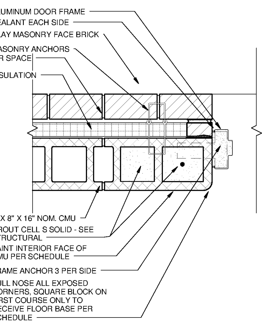
5 DOOR JAMB TYPE A.1 A-3102 SCALE: 1 1/2" = 1'-0"
