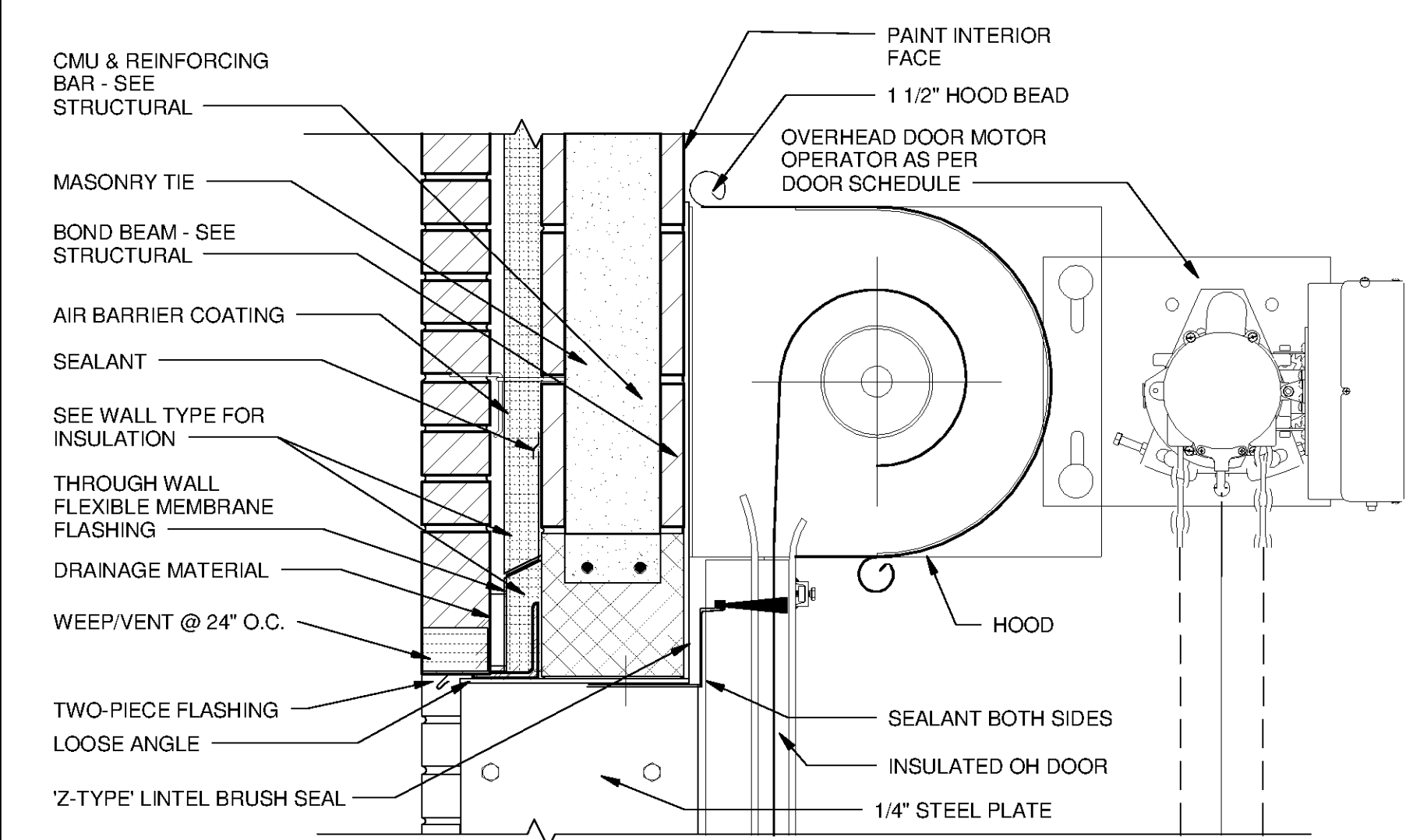
12 DOOR HEAD TYPE OH.1 A-3302 SCALE: 1 1/2" = 1'-0"
