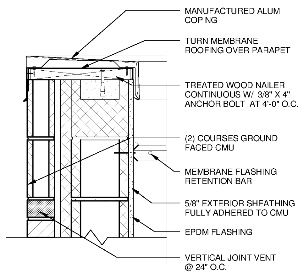
4 PARAPET DETAIL A-3302 SCALE: 1 1/2" = 1'-0"
