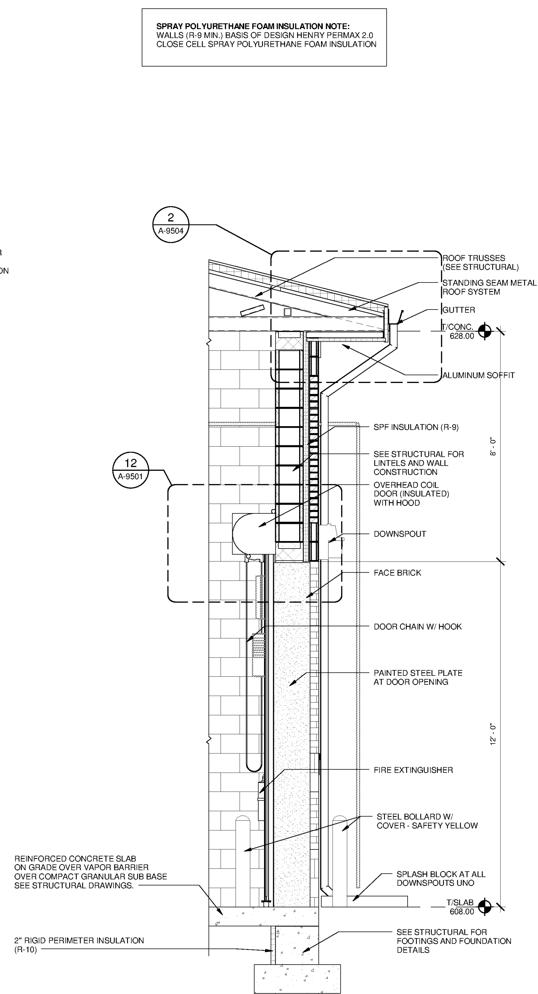
1 WALL SECTION A-3202 SCALE: 1/2" = 1'-0"
