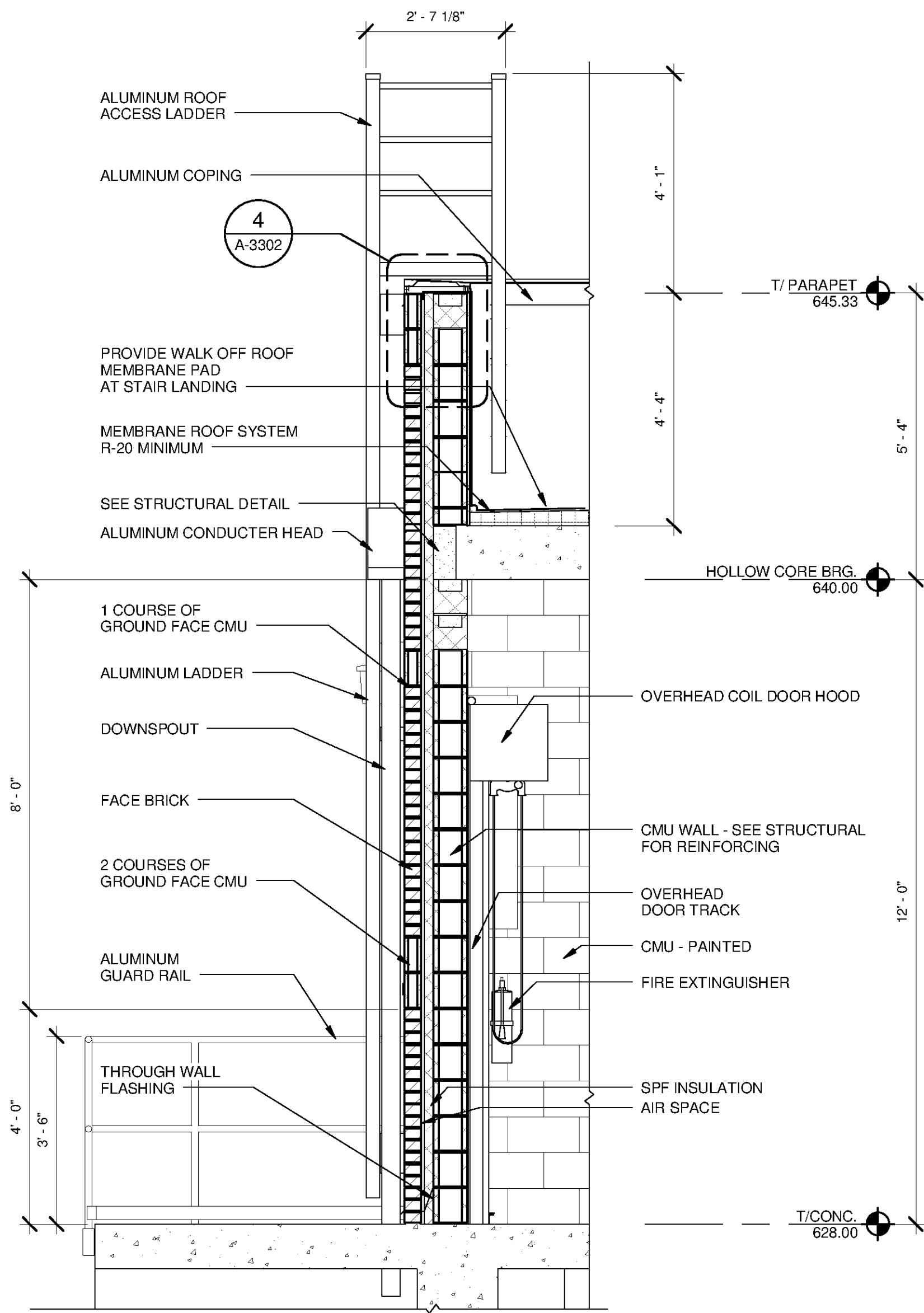
3 WALL SECTION A-3202 SCALE: 1/2" = 1'-0"
