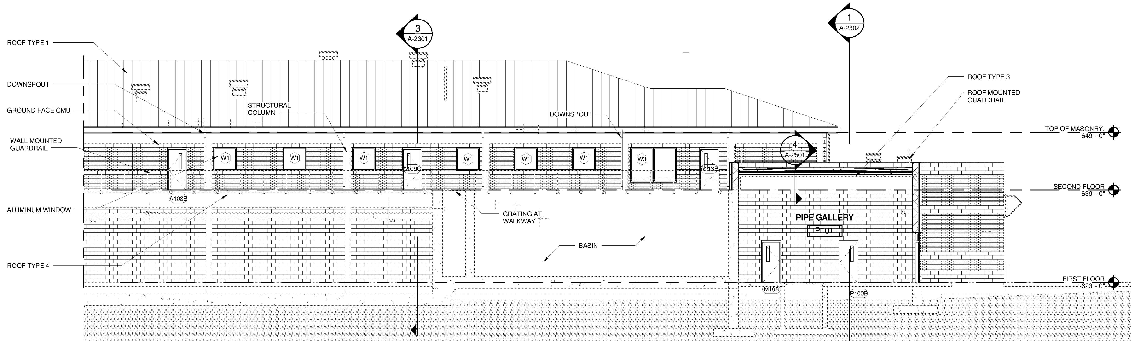
SOUTH ELEVATION - B SCALE: 1/8" = 1'-0"
