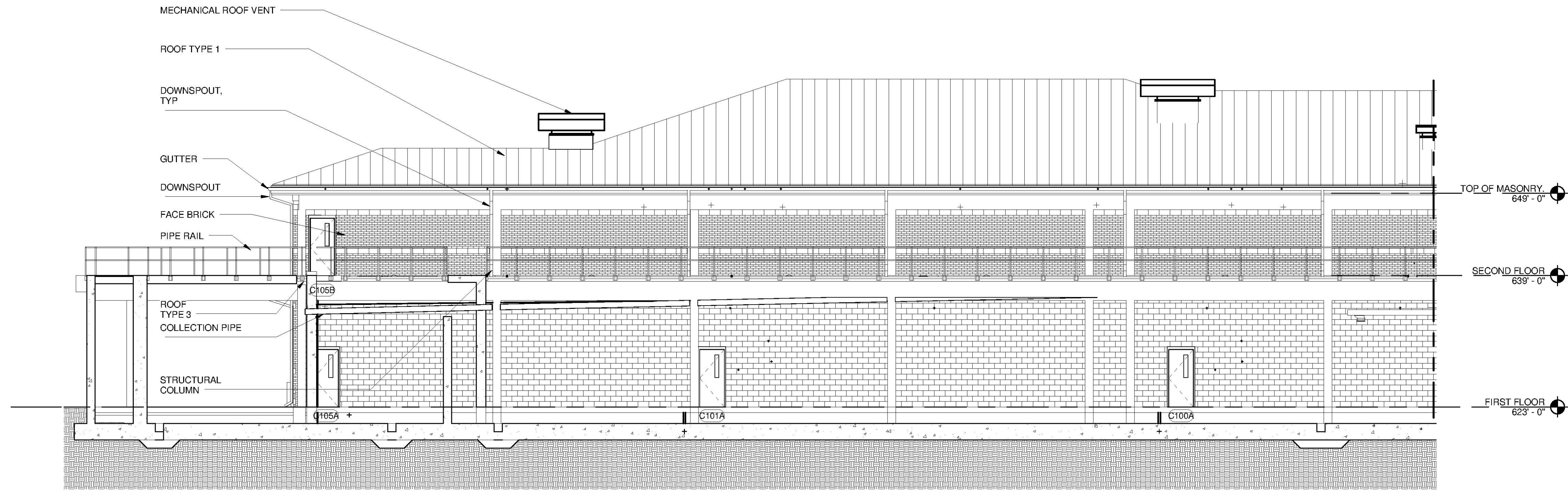
SOUTH ELEVATION - A SCALE: 1/8" = 1'-0"
